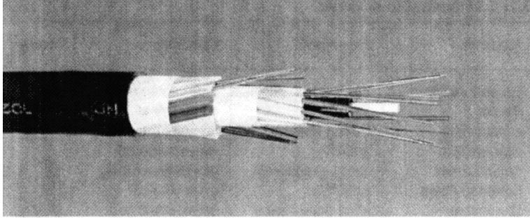
الشكل 3-23 مثال على أنبوب الليف الرخو كثير الألياف (تقدمة شركة براند - ركس)
