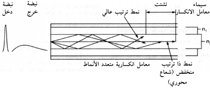
الشكل 17-2 ليف تأشير انكسار متعدد الأنماط.
