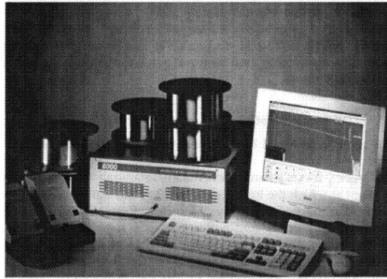
الشكل 8-10 جهاز نيت تست/ بي كي تكنولوجيا نموذج 8000 OTDR (تقدمة نيت تست).
