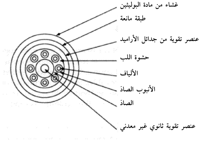
الشكل 3-22 يظهر بنية كابل ليف بصري ذا سعة كبيرة
