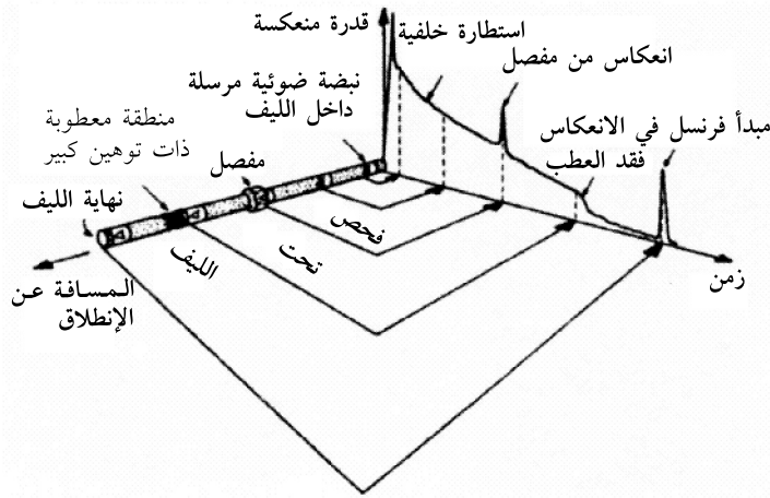
الشكل 8-8 يوضح المبدأ الذي يعمل عليه مقياس الانعكاس لمجال الزمن البصري باستخدام نظرية رايلييه للاستطارة الضوئية لفحص منظومة الليف البصري.
