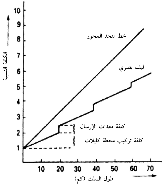
الشكل 3-7 مقارنة بين كلفة النظام متحد المحور وكلفة النظام الليفي البصري لمعدل إرسال بقوة 565 ميغابت في الثانية.
