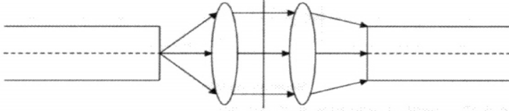
الشكل 15-6 القرن العدسي المتناظر
