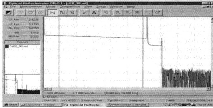
الشكل 8-9 برنامج تعقب خاص للجهاز البصري لقياس انعكاسية المجال الزمني (OTDR)
