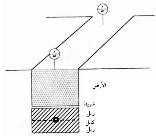
الشكل 7-20 كابل موصد في خندق
