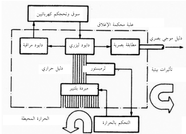
الشكل 4-9 رسم تخطيطي يظهر الصمام الثنائي الليزري المرزوم بإحكام داخل علبة.
