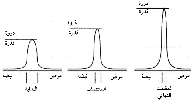
الشكل 9-2 نبضة موجة وحيدة (Soliton) تنتقل عبر الليف البصري التشبتي.
