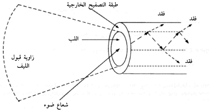
الشكل 2- 14 شعاع ضوء يدخل ليفاً من خارج نطاق زاوية مخروط القبول
