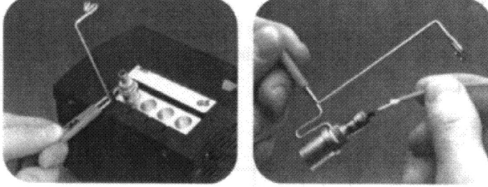
الشكل 6-35 تسخين الأنبوب في سخان أو ملهاف صغير ومن ثم إدخال الليف (تقدمة (AURIGA (Europe) PLC
