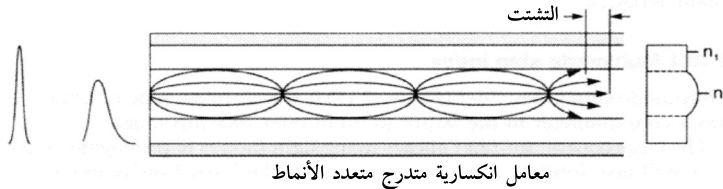
الشكل 18-2 ليف متعدد الأنماط بمعامل انكسار متدرج
