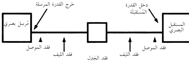
الشكل 7-17 موازنة الفقد في المسلك البصري (Optical Path)
