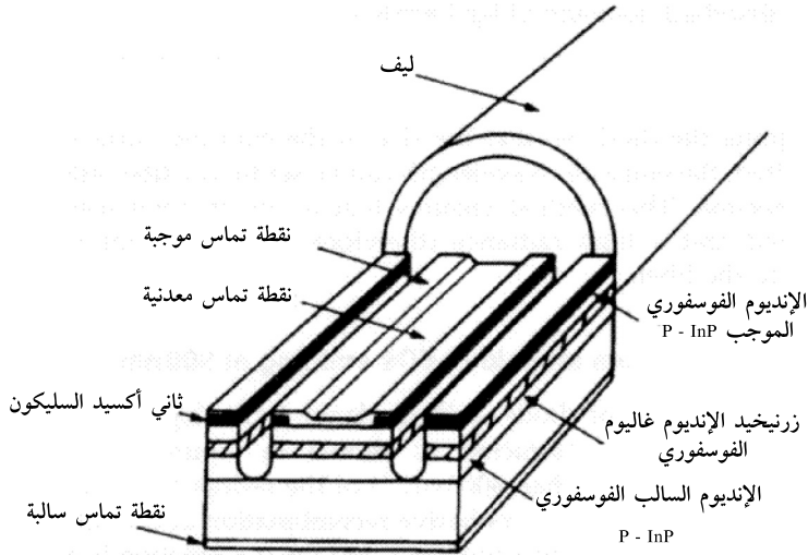
الشكل 4-4 بنية الصمام الثنائي الباعث للضوء من الحافة
