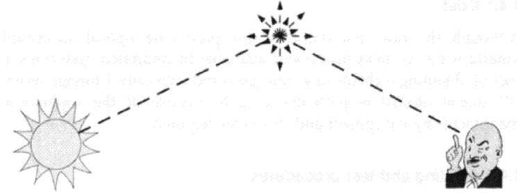
الشكل 1-27 ظاهرة استطارة رايلي (Rayleigh).
