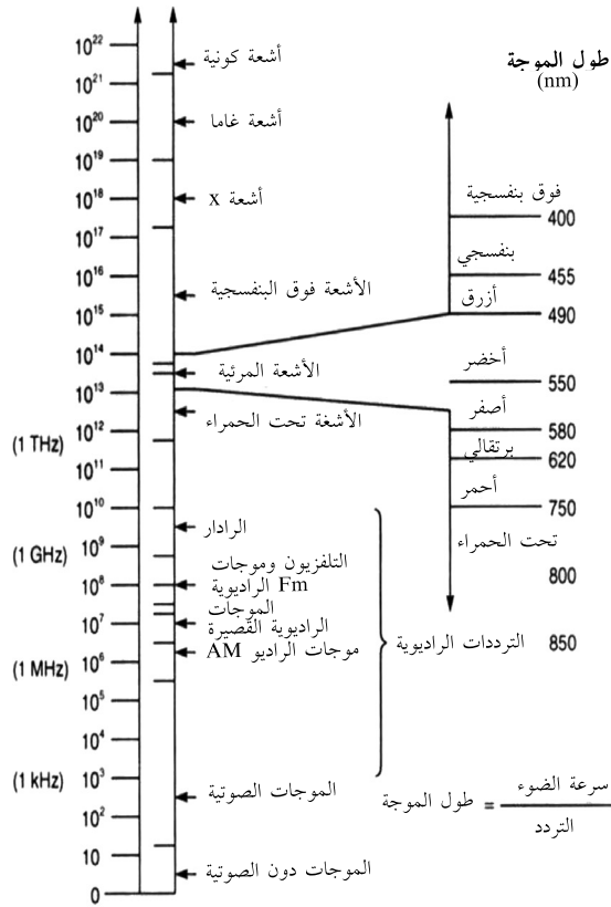
الشكل 20-1 الطيف الكهرومغناطيسي يُظهر أطوال موجات وترددات الإشارات الشائعة (تقدمة : Cable Table Pty Ltd).
