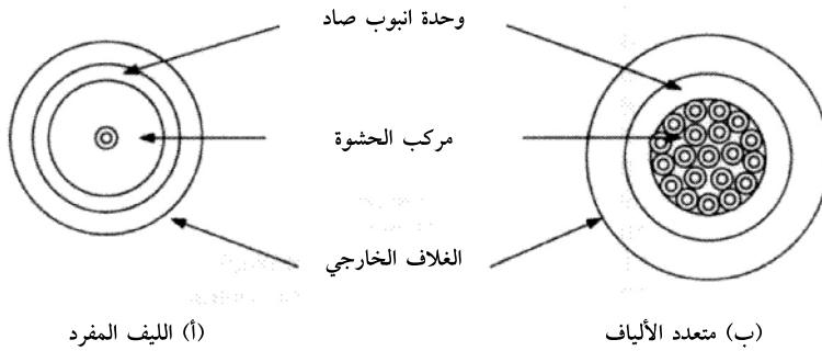
الشكل 3-21 تظهر بنية كابل ليف بصري متوسط السعة
