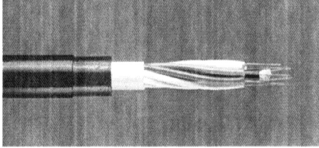
الشكل 3-27 مثال على تصميم كابل أنبوبي مدرع، مجدول غير معدني مع حماية من القوارض (تقدمة بي آي سي سي براند - ريكس)
