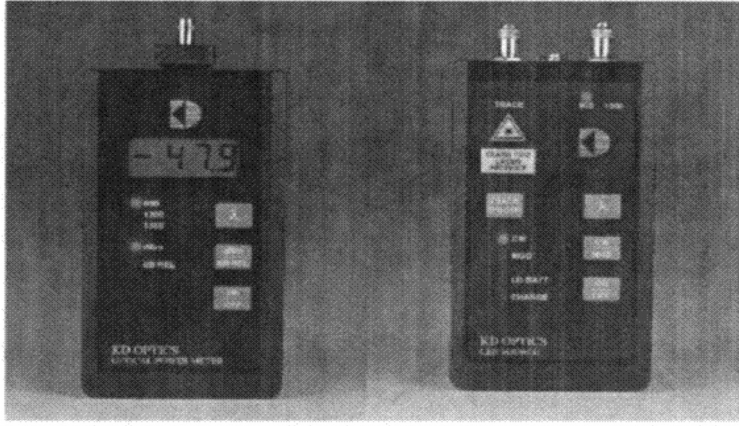
الشكل 7-8 جهاز قياس الطاقة البصرية بي أم 23 (PM23) وجهاز مصدر ضوئي باستخدام الصمام الثنائي الباعث للضوء (LS20DV) (تقدمة كي دي - أوبيكس)
