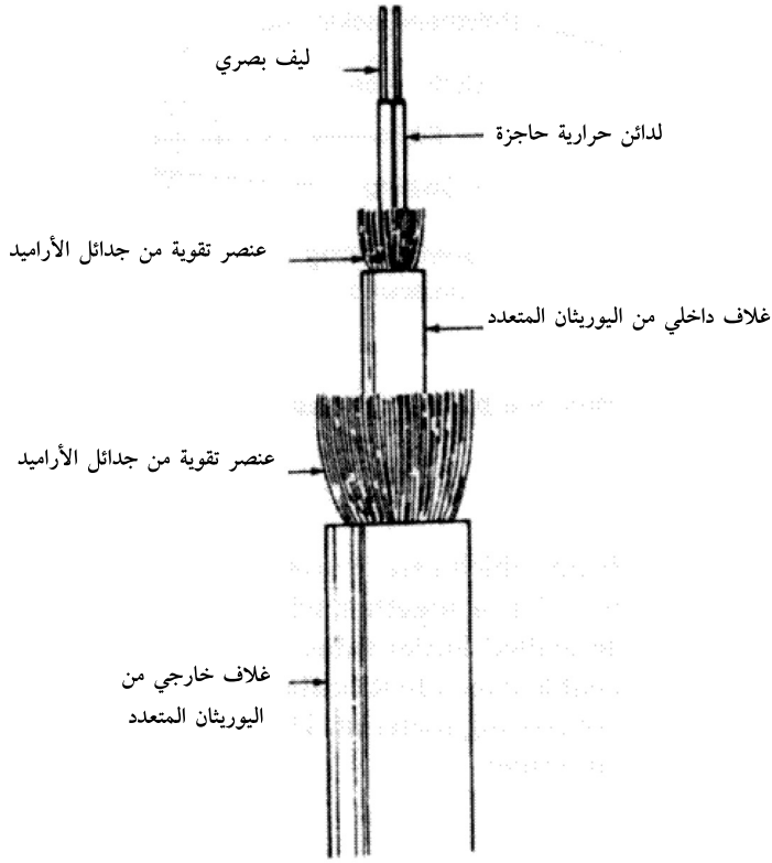
الشكل 3-16 بنية سلك الليف البصري المتعدد الألياف المقوى، والمناسب للبيئات الصعبة (كلاستخدامات العسكرية).
