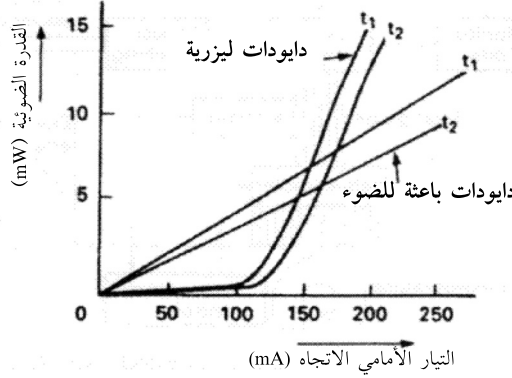
الشكل 3-9 ميزات الطاقة البصرية مقارنة بالتيار الأمامي لليزرات والصمامات الثنائية الباعثة للضوء.
