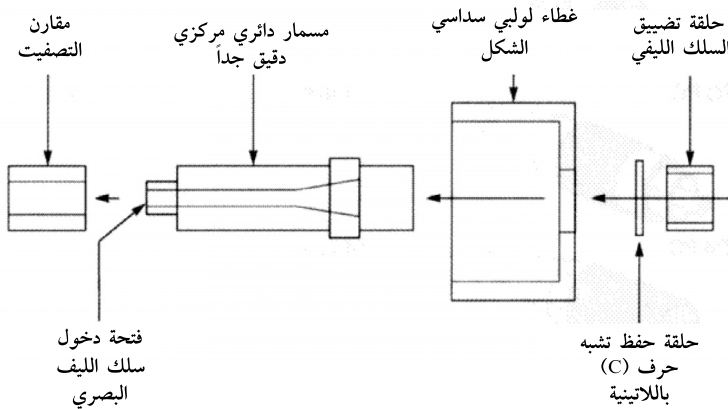
الشكل 2-6 الموصل ذو التجميع المتعدد الثانوي (SMA - Sub Multiple Assembly)
