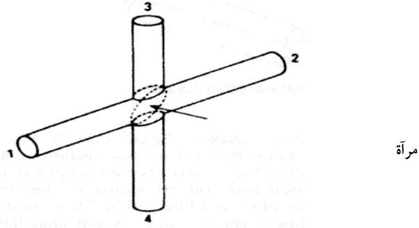
الشكل 6-21 مقرون بأربع فتحات مع مرآة تقسيم (Four-Port With Beam-Splitting Mirror)
