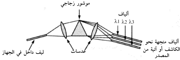
الشكل 2-40 مضاعفة بتقسيم طول الموجة باستعمال الموشور.
