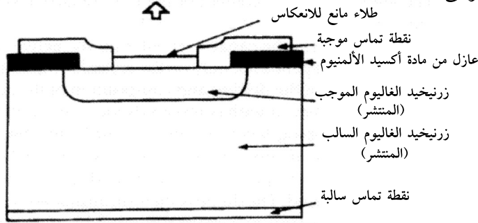
الشكل 4-5 بنية صمام زرنكسيد الغاليوم المنتشر الثنائي الباعث للضوء
