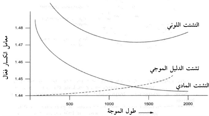
الشكل 2-26 يظهر الرسم البياني «للمعامل الانكسار المؤثر» لليف البصري مقارنة بالطول الموجي للتشتت اللوني والمادي والدليل الموجي.
