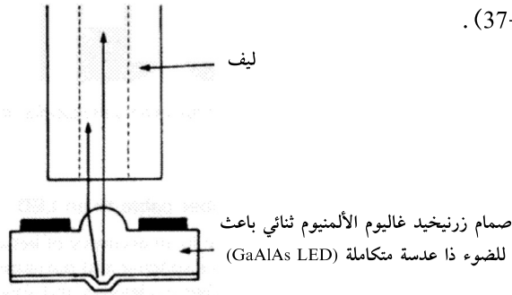
الشكل 37-6 القرن العدسي لليف بصري في صمام ثنائي باعث للضوء
