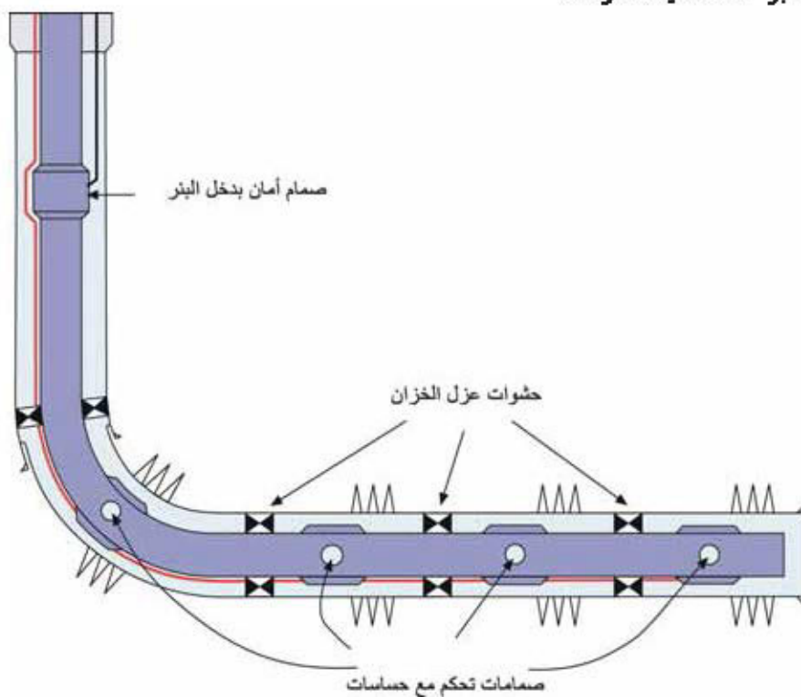
الشكل (10-25) : مثال عن البئر الذكية.
