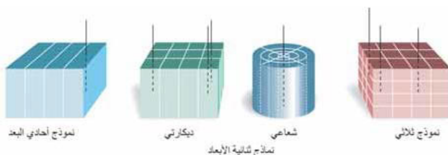
الشكل (9 - 18): أشكال نمطية لمواقع شبكة القياسات من أجل محاكاة الخزّان.
