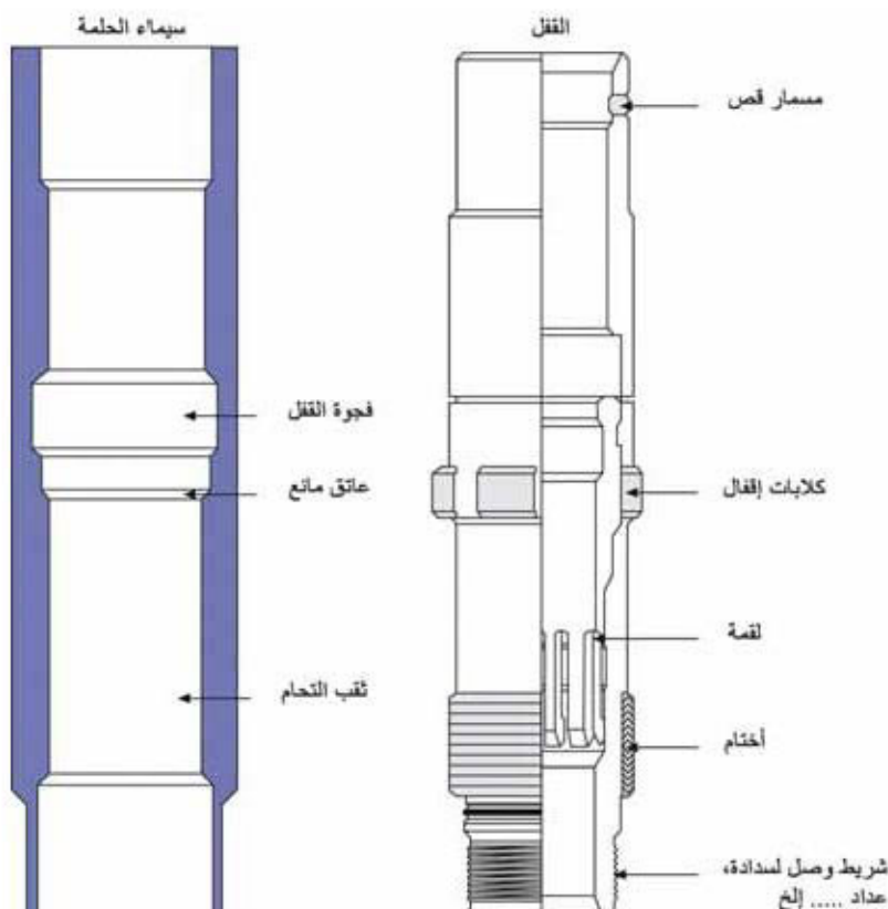
الشكل (10- 24) : مقطع جانبي للحلمة والقفل للرائق.
