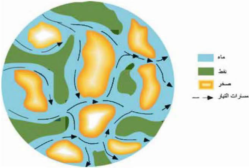
الشكل (6 - 51): مرور التيار الكهربائي عبر الخزآن.
