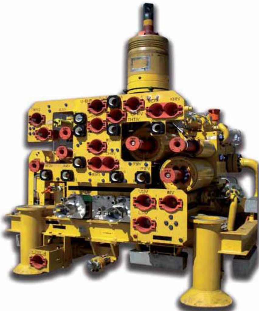
الشكل (10- 32) : شجرة ألفية تحت بحرية (حقوق النشر لـ D. Thomas, 2006).
