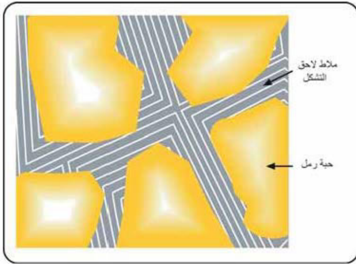
الشكل (6 - 10): تدمير المسامية بالسمنة.
