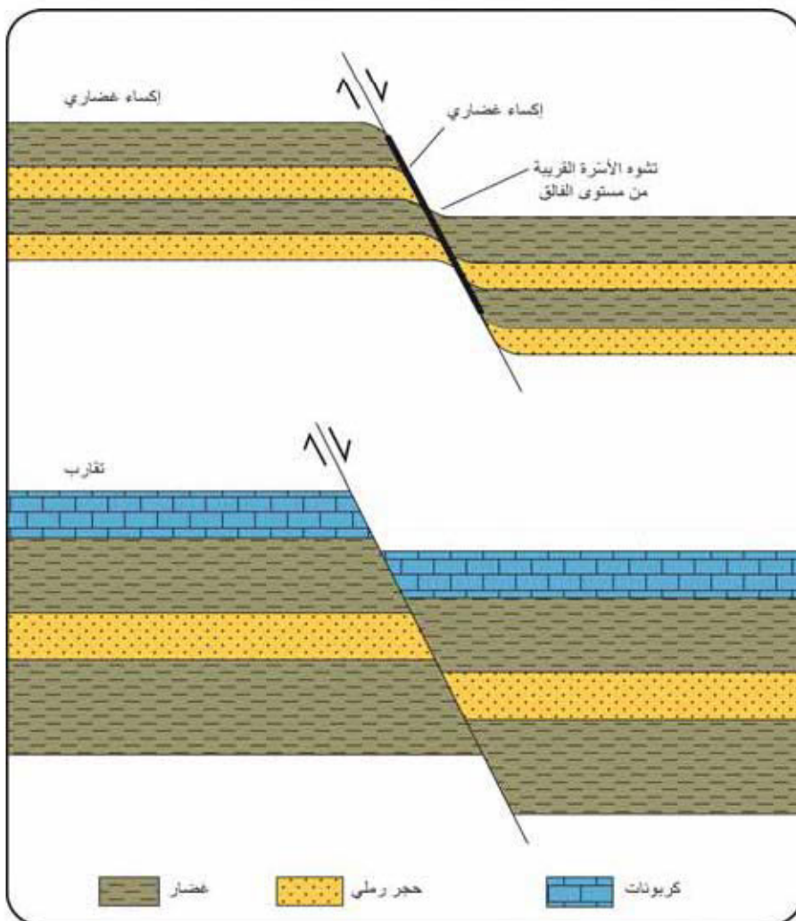
الشكل (6 - 7) : ختم القالِق بواسطة الإكساء بالغضار أو بالتقارب.
