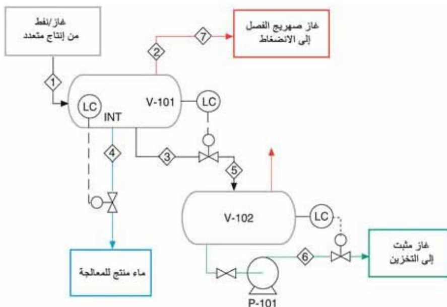
الشكل (11 - 3) : مخطط لتلق العملية الرئيسي (PFS).
