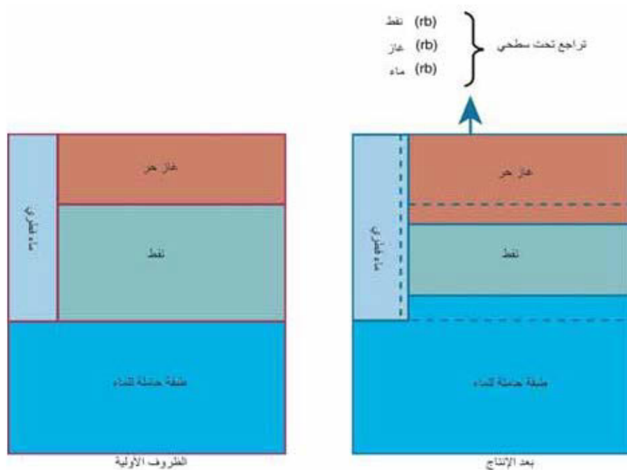
الشكل (9 - 1) : تعدد الموائع لتحل محل الحجم المنتج.
