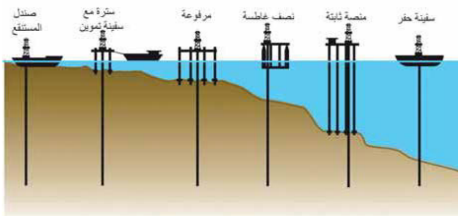
الشكل (4 - 1) : أنواع منصّات الحفر البحرية.
