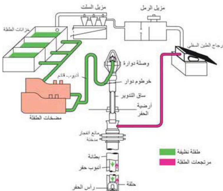
الشكل (4 - 11): منظومة تصوير الطقيلة.
