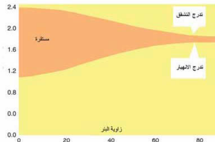
الشكل (4 - 15): مثال عن العلاقة بين وزن الطغلة واستقرار البئر.
