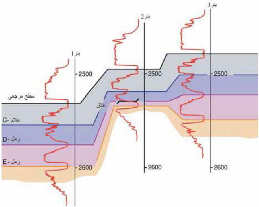
الشكل (6 - 42): لوابط بنيوي.
