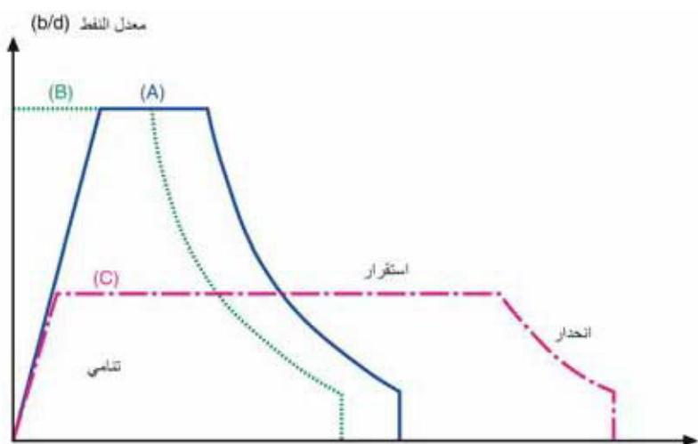
الشكل (9 - 20): منحنيات خطقة لنفس الاستعادة النهائية.
