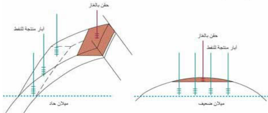
الشكل (9 - 5) : موقع الآبار للسوق بغاز القبة.
