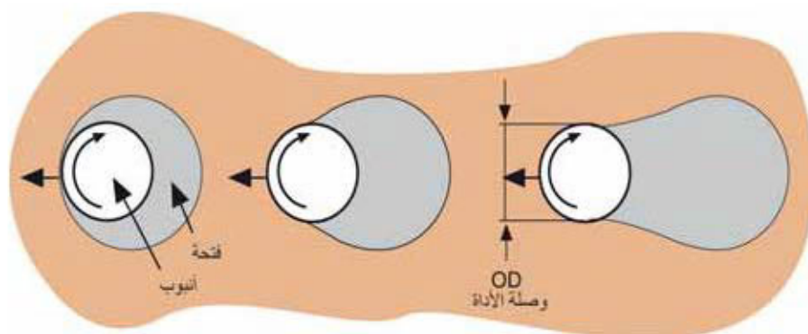
الشكل (4 - 26): تطور إلقاء الفتاح (منظر مسقط أفقي للمحفرة).
