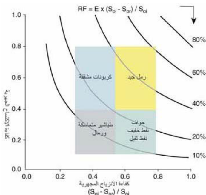
الشكل (9 - 19): تأثير عامل الاستعادة بالتشابه.
