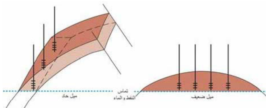
الشكل (9 - 2) : موقع الآبار وأثره في قطع الموائع بالغاز.
