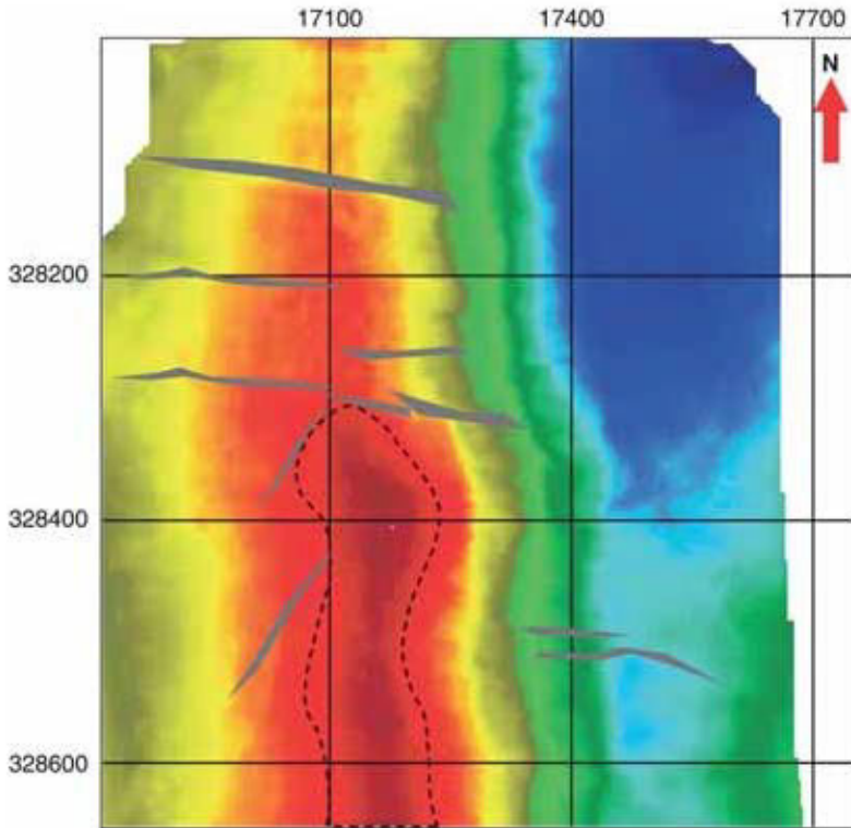
الشكل (3 - 24) : خريطة بنيوية سطوية مع تعيين الفوالق والمحتوى الهيدروكربوني (الخط المتقطع).
