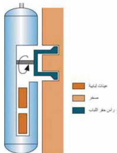
الشكل (6 - 35): أداة حفر العينة اللينة الجدارية.
