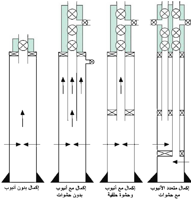
الشكل (10 - 20) : ملخص أشكال الأنبوب.
