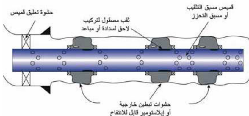
الشكل (10-17) : إكمال بئر مفتوحة (open hole) مع عزل نظائلي.
