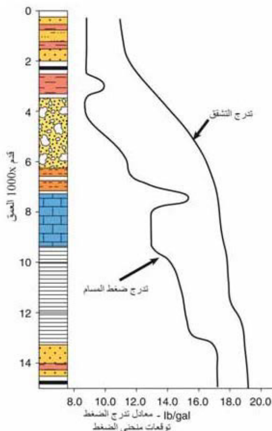
الشكل (4 - 14): يجب أن يكون غلاف وزن الطّقة بين تدرج ضغط المسام وتدرج التشقق.
