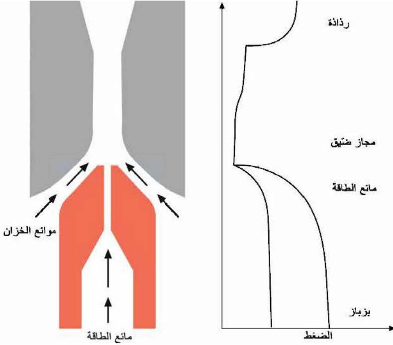
الشكل (10-30): مضخة نفّاثة.
