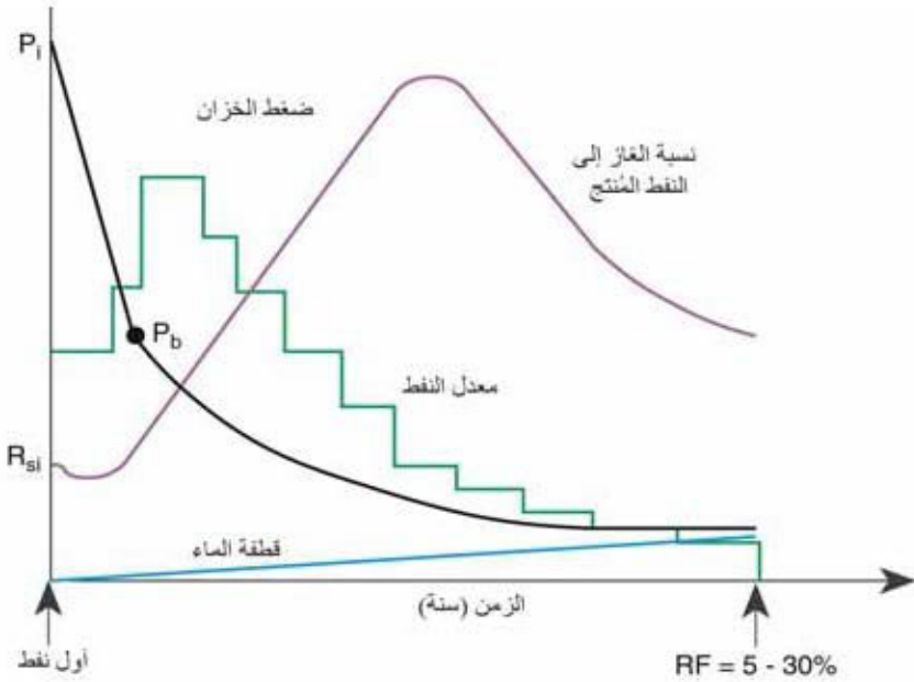
الشكل (9 - 3) : منحنى سيماء الإنتاج لحِزْن يُساق فيه المائع بالغاز (حقن غازي).
