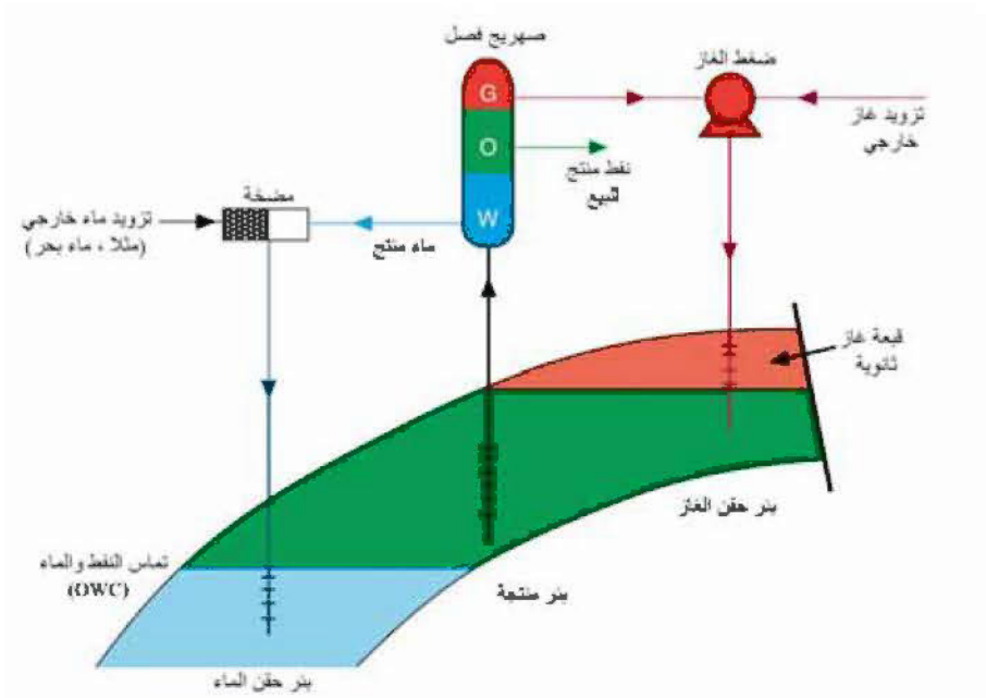
الشكل (9 - 4) : الاستعادة الثانوية: مشروع حقن غاز أو ماء.
