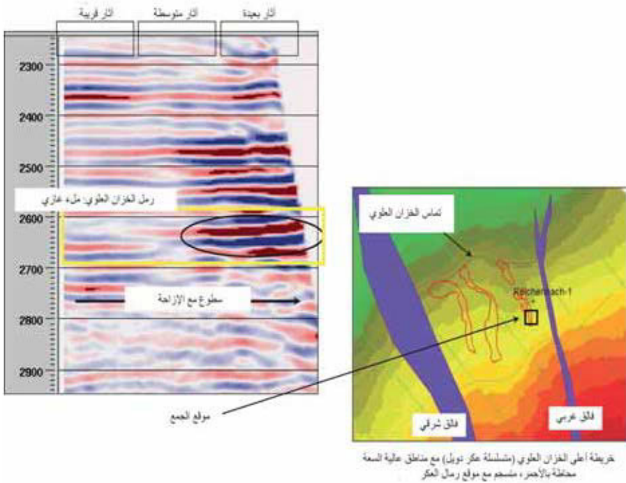
الشكل (3 - 27) : تنتج الرمال الممتلئة بالغاز في سلسلة دويل Doyle الكنتية (الحفران العلوي) سمات سيمية لزيادة بازدياد التباين.
