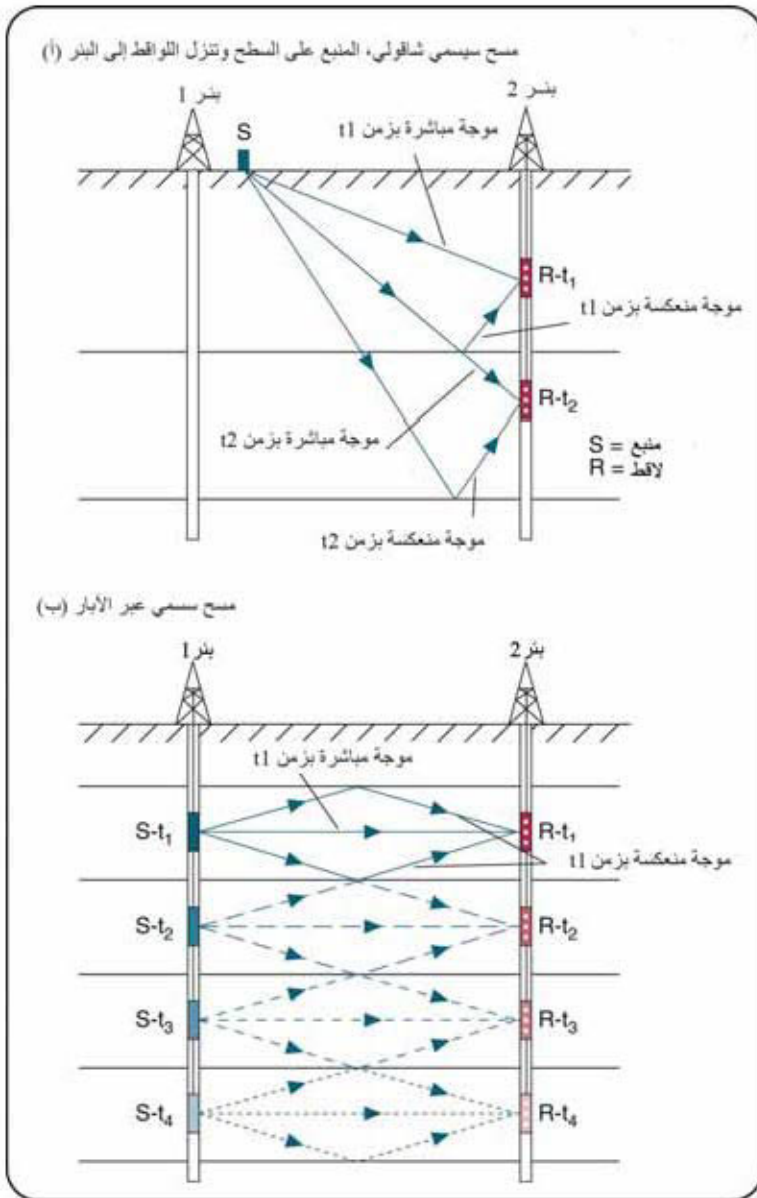
الشكل (3 - 17): مبدأ المسح السيزمي البئر.
