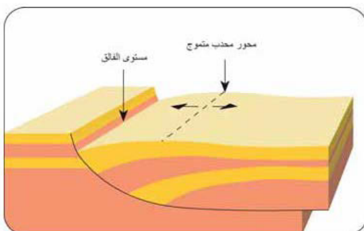
الشكل (6 - 6) : هندسة تصدع النمو والمحدب الناتج (متموج rollover) (من بتروليوم هانديوك 1983).
