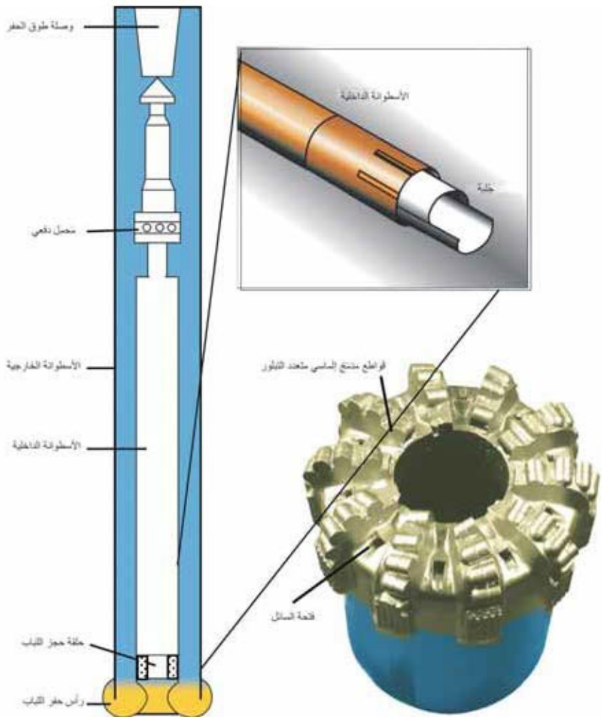
الشكل (6 - 32): تجميع جهاز اعتيان اللباب ورأس حفر اللباب (يأخذ من Security DBS (abd Corepro).
