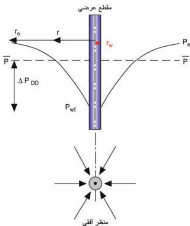
الشكل (10-2) : توزيع الضغط حول البئر.
