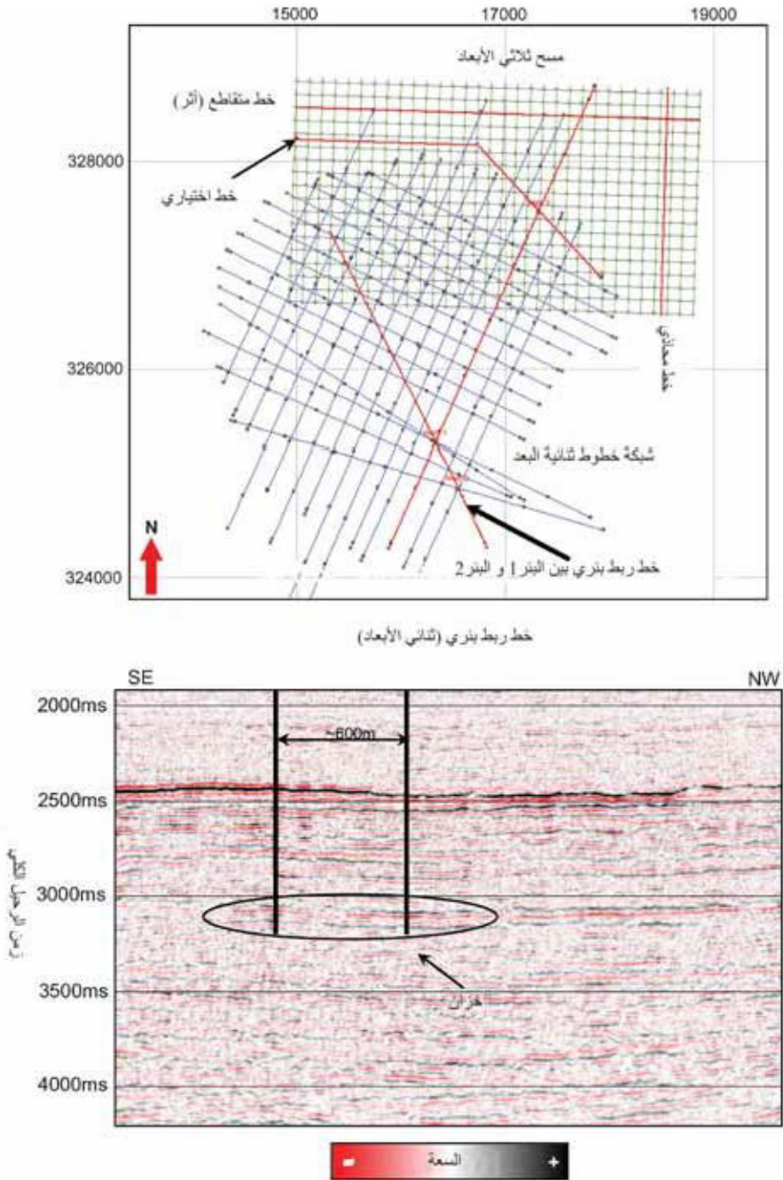
الشكل (3 - 22): خريطة التركيزية مع شبكة خطوط مسح ثنائية البعد ومسح ثلاثي الأبعاد (شكل علوي)، وخط ربط بنري ثنائي البعد في مقطع شاتوبلي (شكل سفلي).
