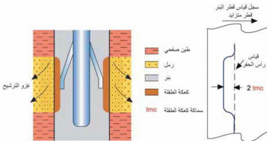
الشكل (6 - 55): قياس سمكة الطفلية.
