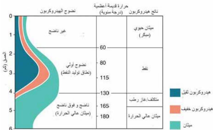
الشكل (3 - 4): نضج الهيدروكربون.
