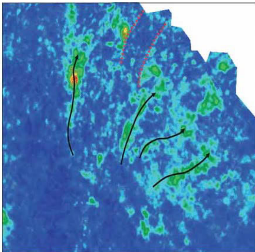
الشكل (3 - 26) : خريطة ستراتغرافية : تشير السمات البراقة (أخضر ، أصفر ، أحمر) إلى وجود آنية عكر ، لاحظ تأثير التصدع (الخط الأحمر للقطع) في نقل الرسوبيات (الأسهم).
