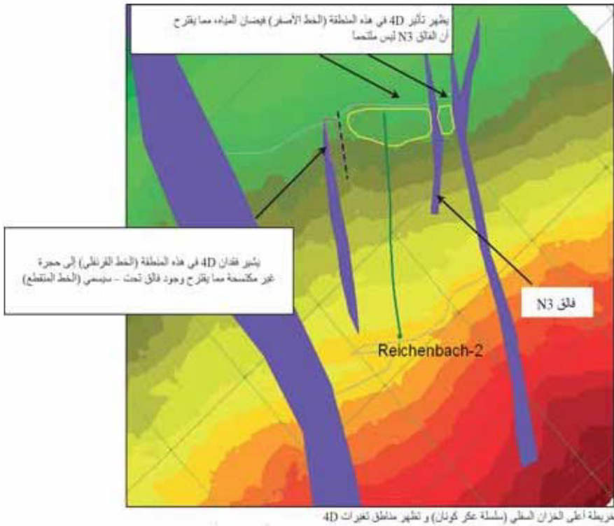
الشكل (3 - 29): تتبّع حركات تماس الموائع باستخدام المعطيات السيسمية وباهية الأبعاد.
