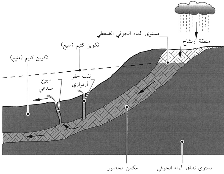
الشكل 8: ينبوع صدعي أرتوازي وثقب حفر أرتوازي. المصدر: WEDC.
