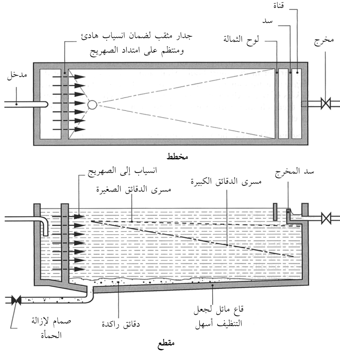
صهريج تركيد بسيط. المصدر: WEDC.
