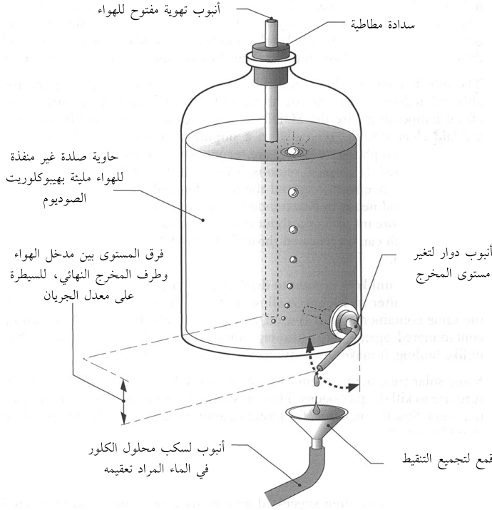
سفافة الرأس الثابت. المصدر: WEDC.
