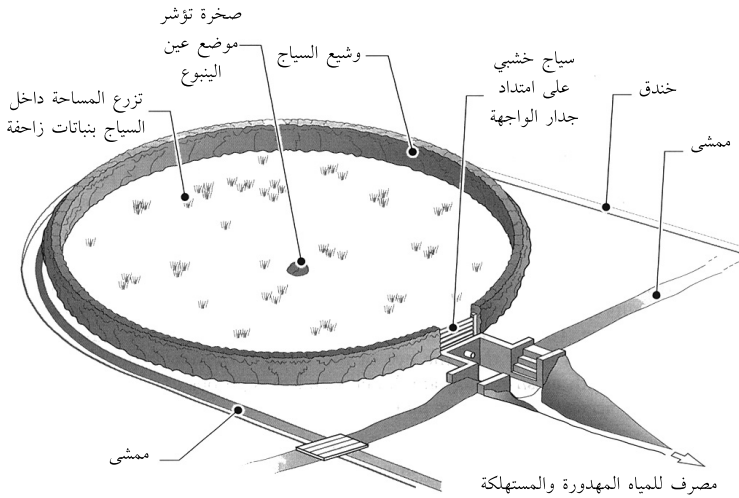
الينبوع بعد اكتمال جهوزيته. المصدر: Shaw (1999).
