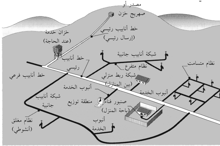
مستوى التأسيس الذي يشكل نظام شبكة التوزيع. المصدر : WEDC .
