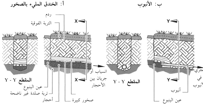
طريقتان لتحصيل الماء ونقله من عين الينبوع. المصدر: Shaw (1999).
