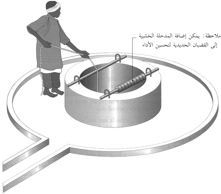
ملاحظة: يمكن إضافة المدحلة الخشبية إلى القضبان الحديدية لتحسين الأداء المصدر: WEDC .
