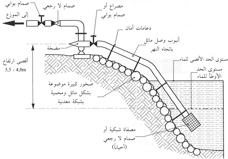
مسرب مص ثابت مع مضخة آلية . المصدر: (Pickford 1991).
