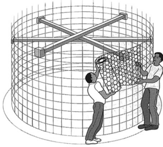
1. أفراد شبكة معدنية مُلحَمة ثم صبها في الأرضية، يضاف مشبك أقفاص الدجاج وأسلاك حلزونية إلى الخارج للتعوية
