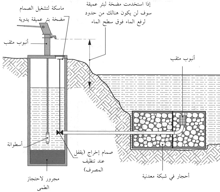
مسرب ثقالي ثابت مع مجري ومضخة يدوية.
