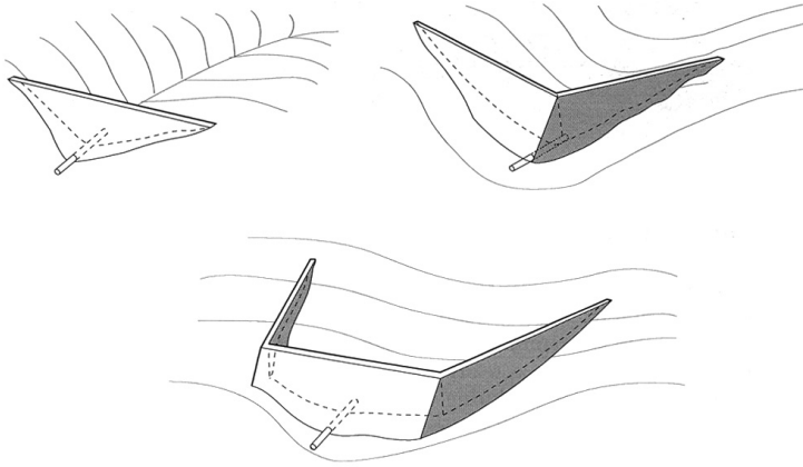
الشكل 52: تكوينات مختلفة لجدران سد مبني من صخور ليخزن ويثبت الصخر. المصدر: Nissen-petersen and Lee (1990).
