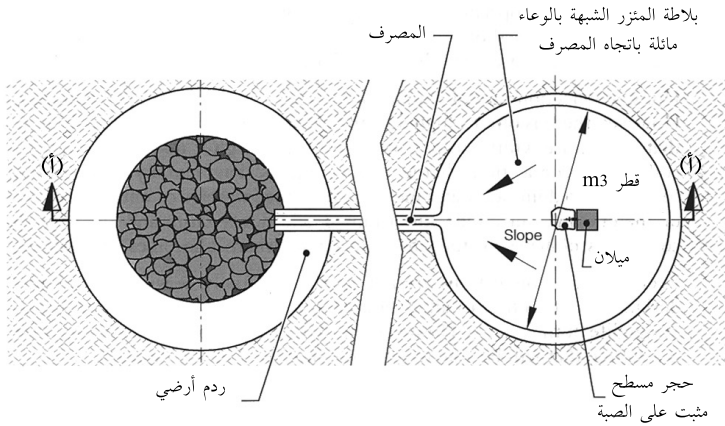
مثال لنقرة نقع مليئة بالصخر تستخدم لتصريف الماء في نقطة توزيع عمومية. المصدر: (DLVW (1983
