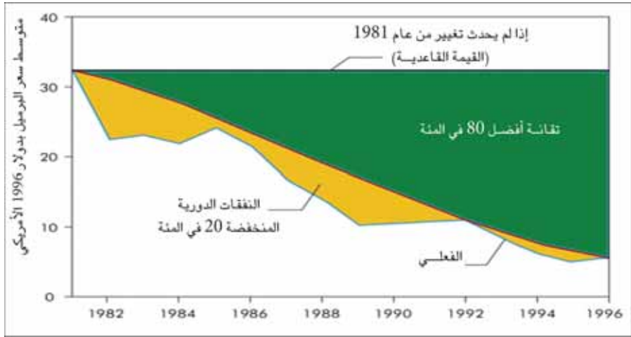
الشكل (2 - 5): تأثير التقانة في الكلفة في مياه الولايات المتحدة
