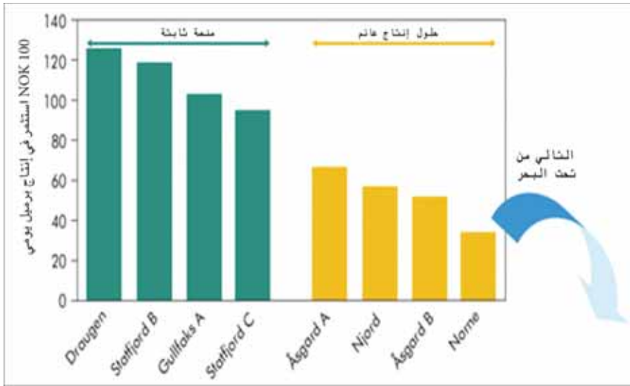
الشكل (2 - 24): تأثير كلفة تطور التقانة بعيداً عن الشاطئ في القطاع النرويجي لبحر الشمال
