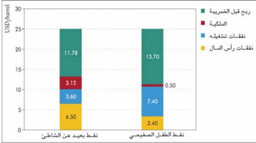
الشكل (3 - 7): بنية كلفة مشروع طّفّل ستوارت النفطي المقترح في أستراليا
