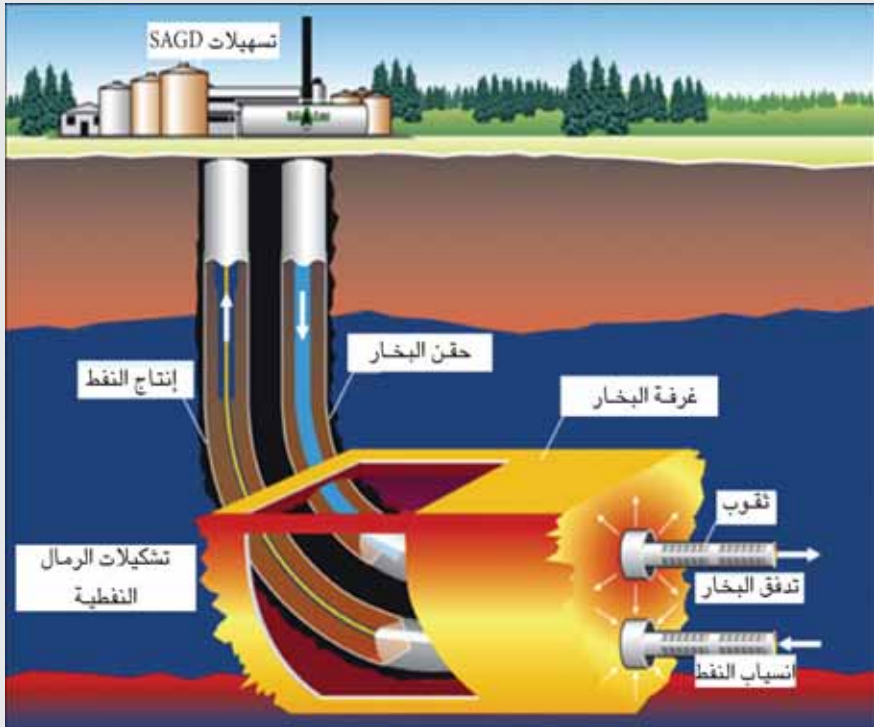
الشكل (3 - 4): عرض تخطيطي لتصريف الجاذبية بمساعدة البخار
