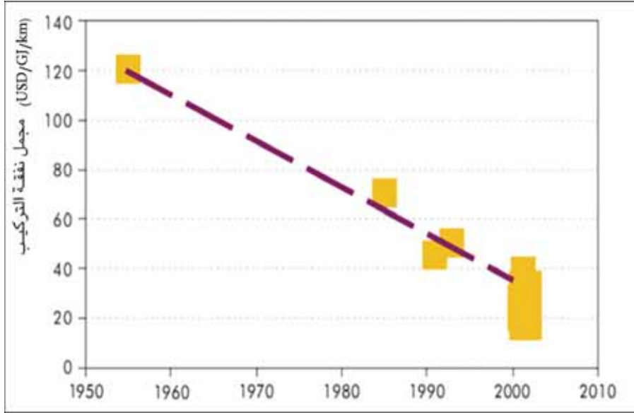
الشكل (5 - 4): تطور كلفة رأس المال لمنشآت تسيليل الغاز بالدولار الأميركي لكل برميل يومياً
