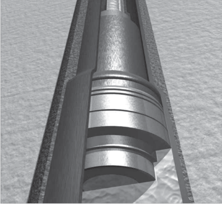
الشكل (2 - 7): خطط للتغليف (أزرق) وسّع بواسطة آلة توسيع سحبت من الأسفل إلى الأعلى
