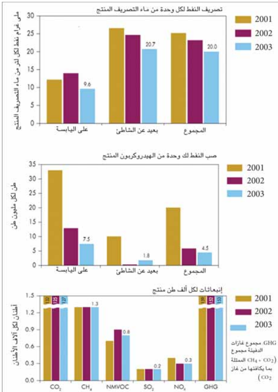
الشكل (6 - 3): اتجاهات في مؤشرات التأثير البيئي الرئيس
