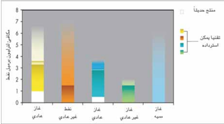
الشكل (1-5): موارد الهيدروكربون في العالم
