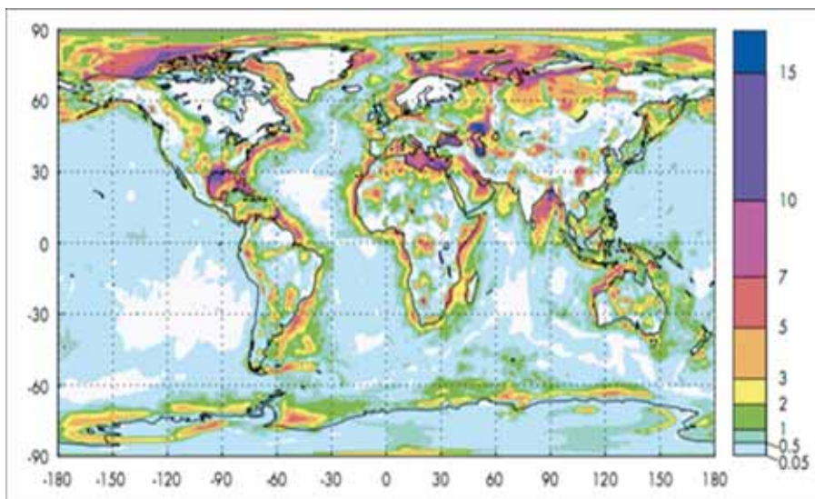
الشكل (2 - 30): خريطة لسماكات الرسوبيات بالكيلومتر
