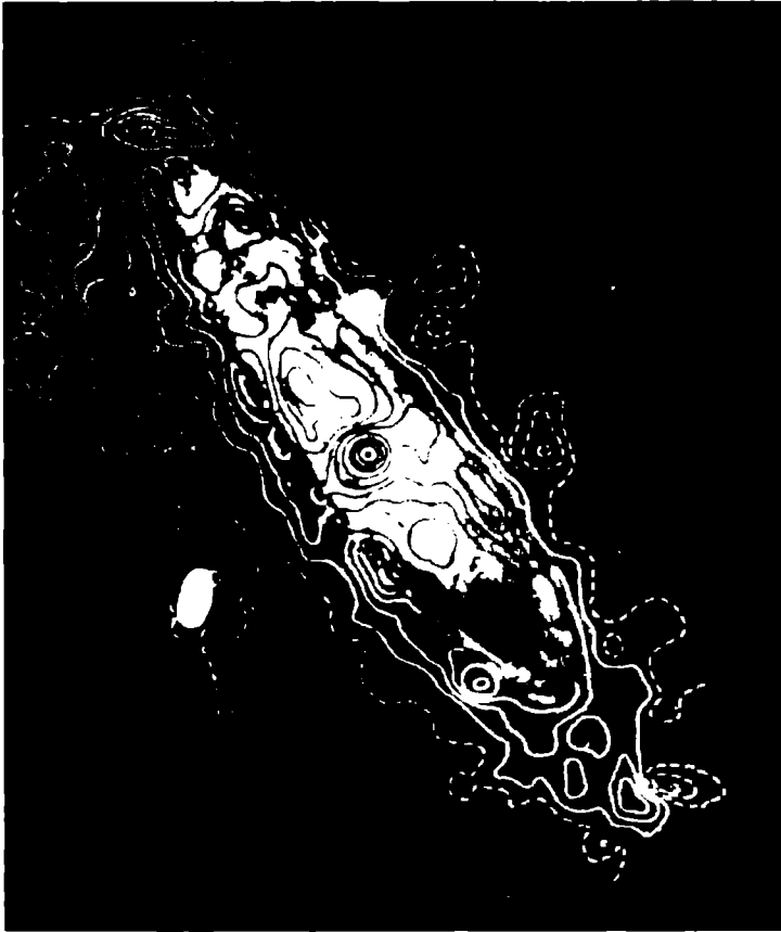
الشكل (47): خريطة راديوية لمجرة أندروميدا غند MH2 408 محملة على صورة بصرية (عن: W. Sciama, Modern Cosmology, 1971).
