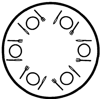
Symétrie de rotation (en faisant tourner l'image six fois d'un « cran », on revient à la position initiale)
