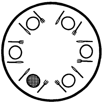
« Rupture » de la symétrie de rotation (le fait d'échanger un couteau et une fourchette rompt la symétrie)
