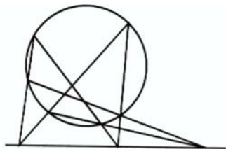
Fig. 5.3 – L'Hexagramme mystique de Pascal
