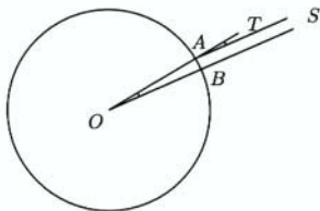
Fig. 2.2 – La mesure d'Ératosthène
