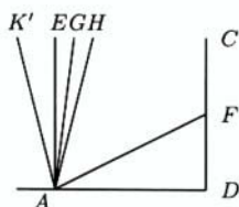
Fig. 8.5 – La parallèle comme coupure.
