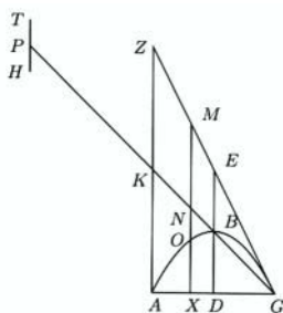
Fig. 2.3 – Méthode de pesée d'Archimède
