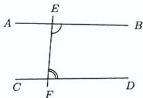
Fig. 2.1 – Postulat d'Euclide
