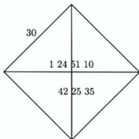
Fig.1.2 – YBC 7289 : \sqrt{2} Crédit : Yale Babylonian Collection
