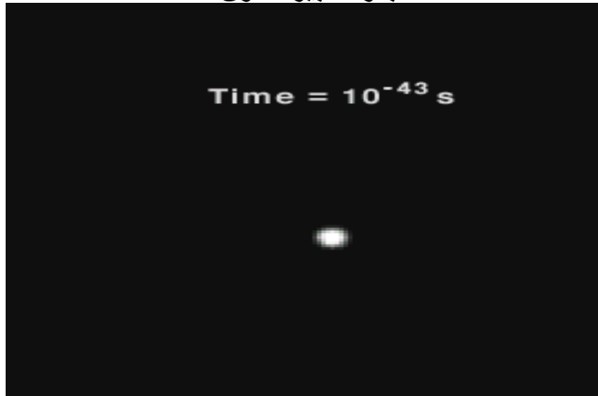
لحظة الانفجار الكبير للكون
