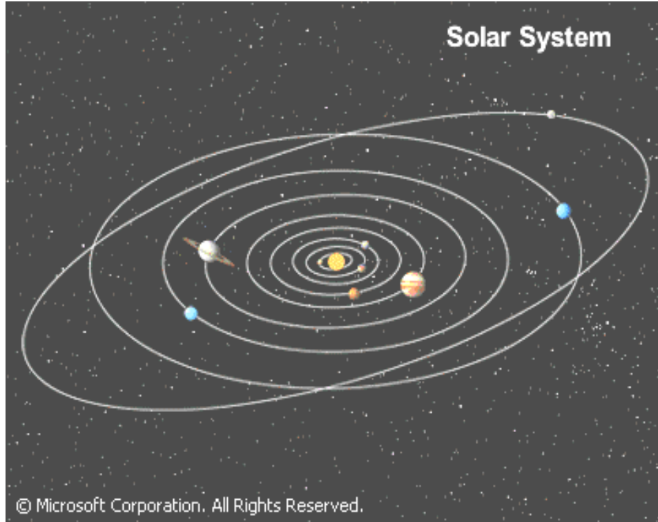
النظام الشمسي
