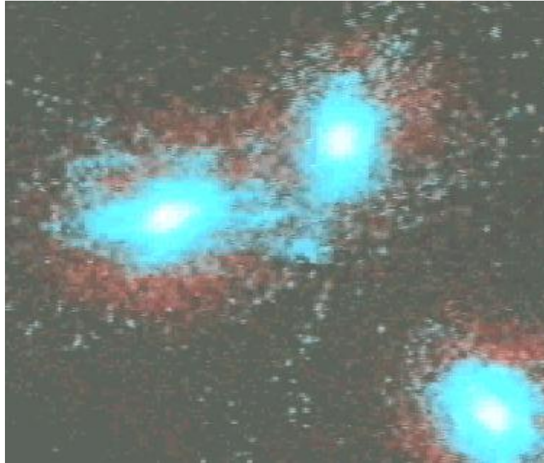
بدء تشكل المجرات
