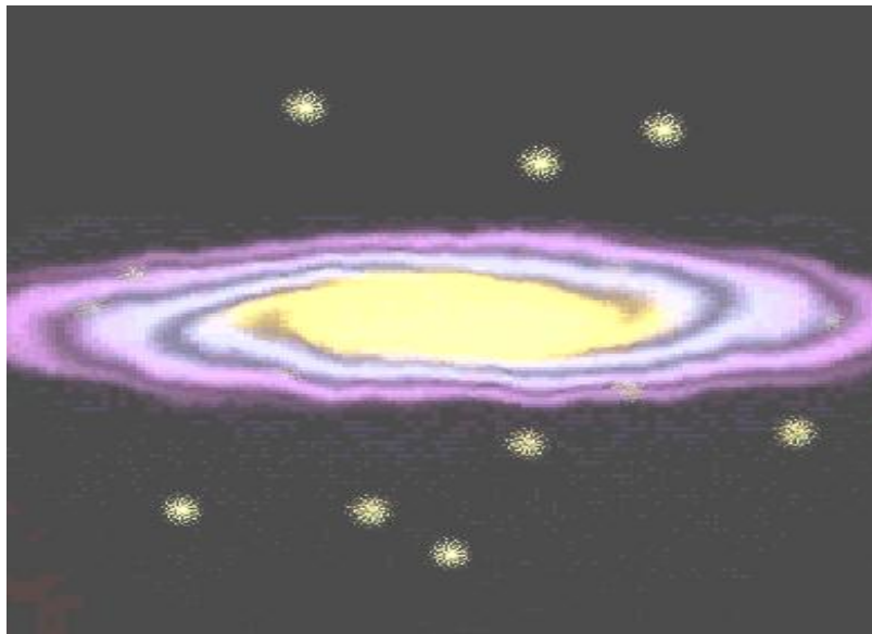
انتظام المجرات وبدء تشكل النجوم
