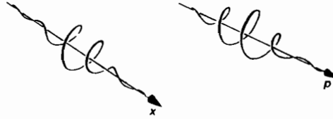
الشكل 6-14: الحزم الموجية المتموضعة في كل من فضاء المواضع وفضاء الاندفاعات.
