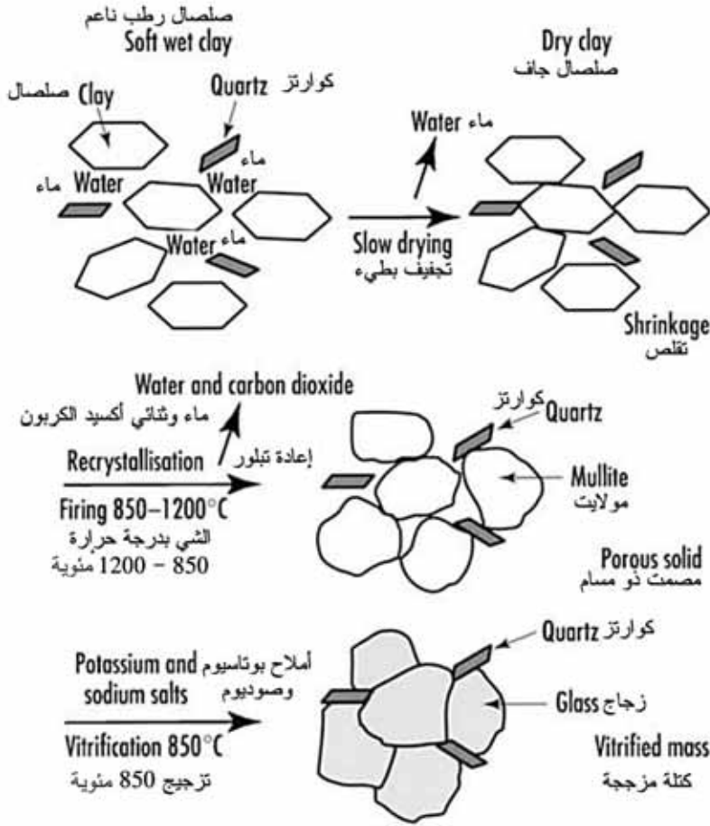
(الشكل 3.8) شبي الصلصال .
