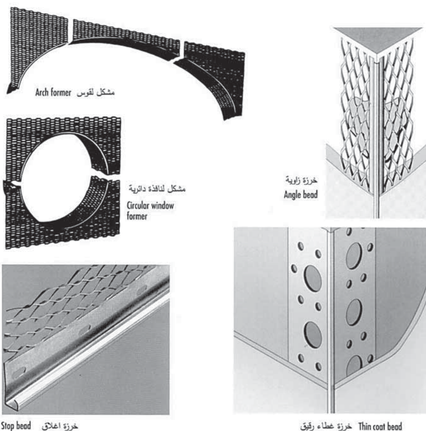
(الشكل 1.12) خرزات الطينة والمشكّلات القوسية.
