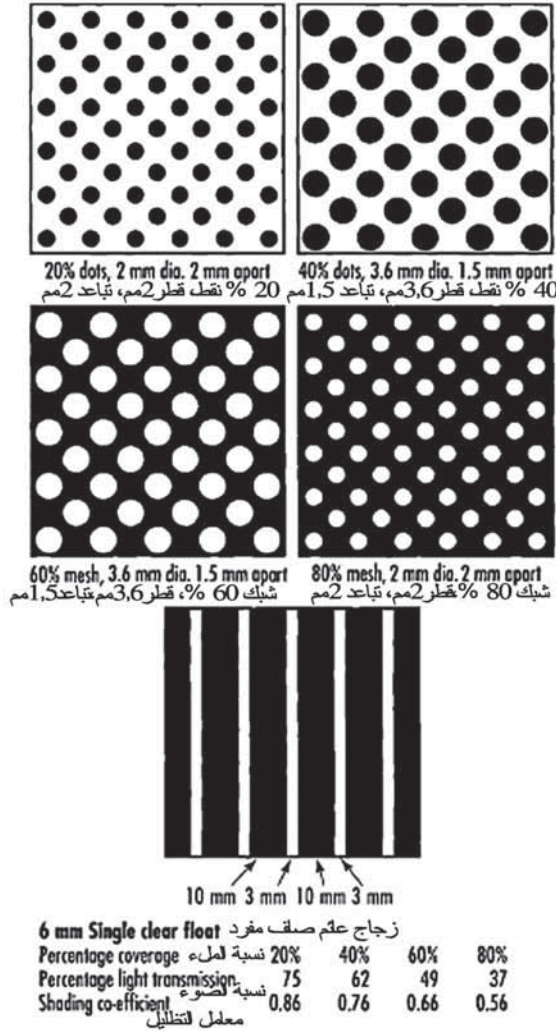
(الشكل 7.7) مختارات من الزجاج النمط (ذي النسيج) مع عامل التغطية المناسب.
