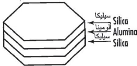
بنية رقائق الإيلايت أو المونتموريلونايت
