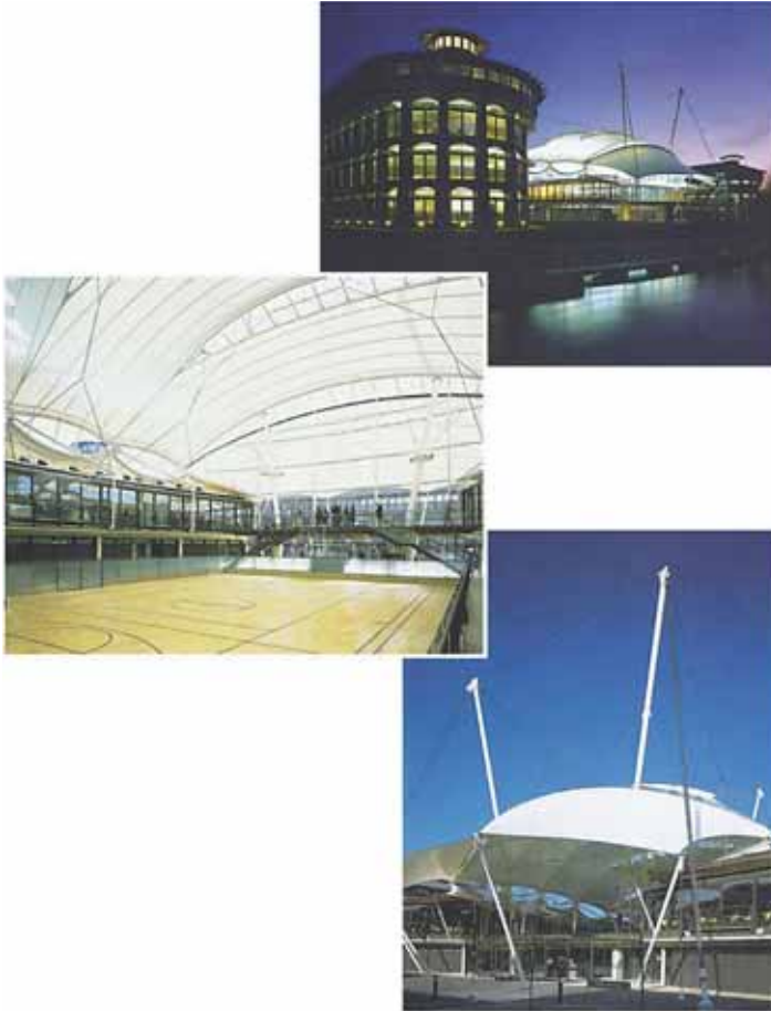
(الشكل 13.10) غشاء الشد - مبنى خدمات الإيرادات الوطنية في نوتنغهام المعماريون: (Hopkins Architects). الصورة بإذن: (MartineHamilton Knight).
