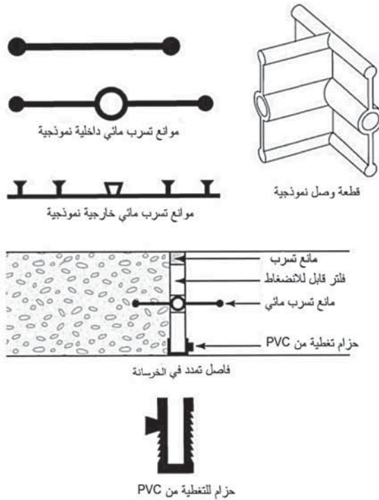
(الشكل 5.14) موانع تسرب الماء في الخرسانة.
