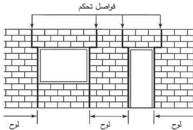
(الشكل 12.2) فواصل الحركة في أشغال البلوك
