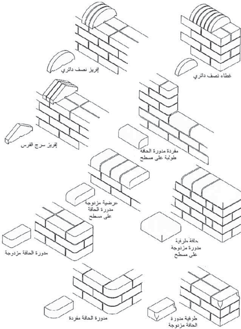
(الشكل 9.1) أنماط الآجر الخاص. الصورة بإذن إيبستوك للآجر.
