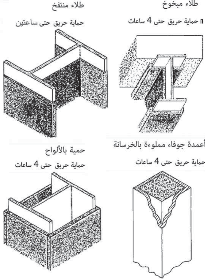
(الشكل 12.5) أشغال الفولاذ البنوي، نظم نموذجية للحماية من الحريق.
