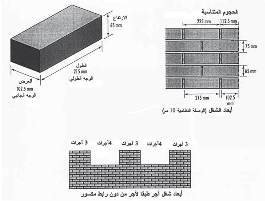
(الشكل 2.1) الأجر والمقاسات المتناسقة.
