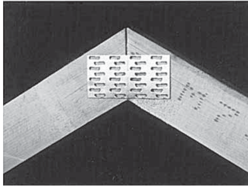
(الشكل 24.4) الصفائح المسمارية.
