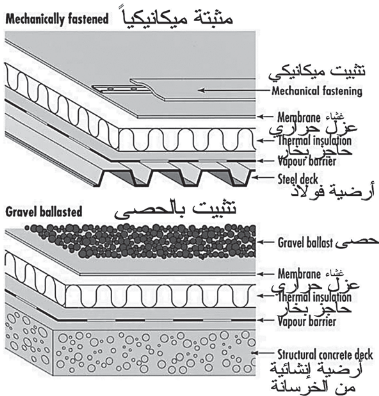
(الشكل 6.6) أنظمة تقليدية وحيدة الطبقة لتغطية السطح، مثبتة ميكانيكياً وفرشة من الحصى.
