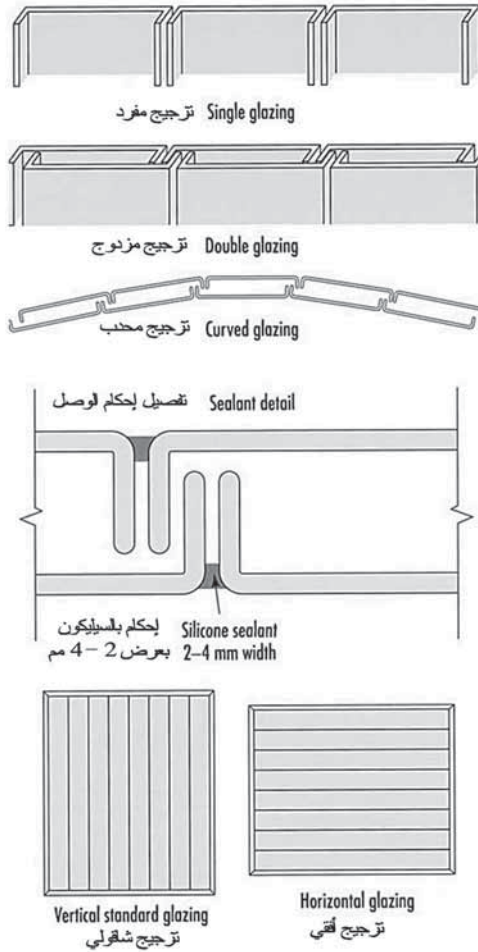
(الشكل 4.7) مقاطع زجاج مكثف الشكل.
