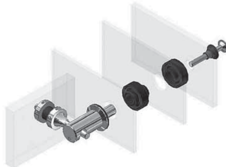
(الشكل 25.7) خطط نظام تزجيج ثلاثي، مقدمة من بيلكينغتون.
