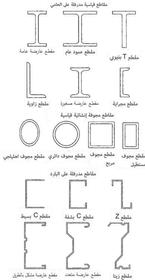
(الشكل 7.5) المقاطع المدرفلة على الساخن والبارد (بعد 1994 Trebilock).
