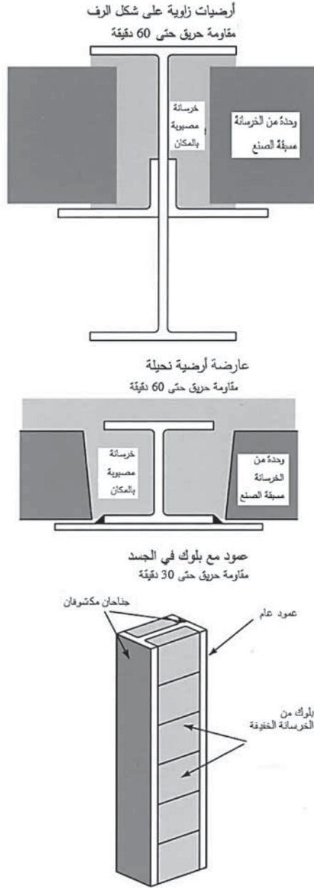
(الشكل 14.5) مقاومة النظم الفولاذية البنوية للحريق .
