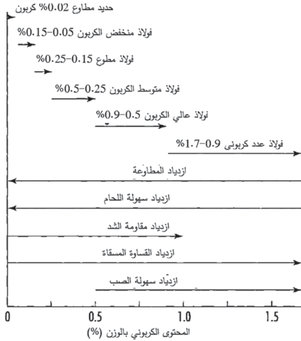
(الشكل 8.5) تأثير محتوى الكربون في خصائص الحديد المطاوع والفولاذ.
