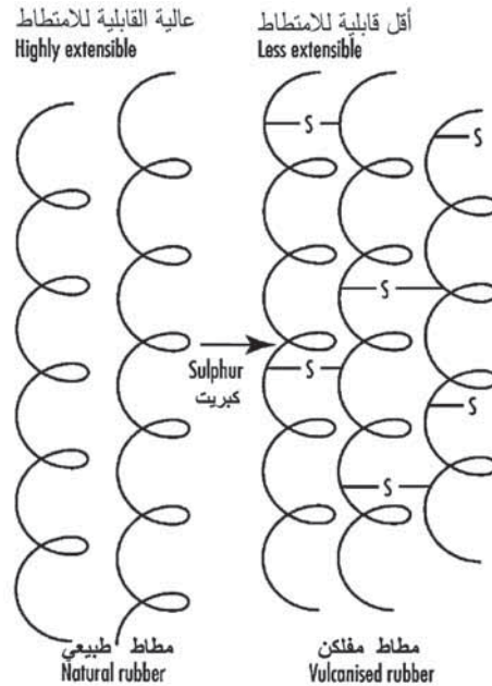
(الشكل 8.10) المطاطيات وتأثير التصليب (التشبيك).
