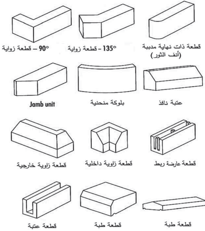
(الشكل 6.2) القطع الخاصة.
