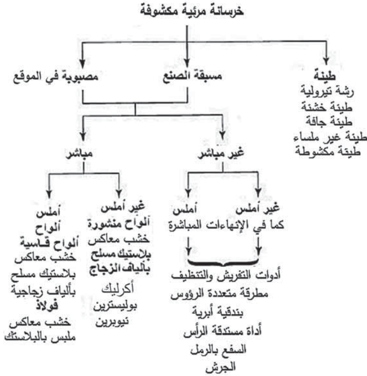
(الشكل 19.3) أنواع الخرسانة البصرية وفقاً للقالب ومعالجة السطح.
