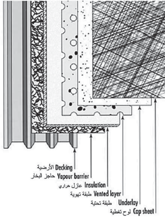
(الشكل 2.6) غشاء القار المسلح التقليدي على نظم السطح.
