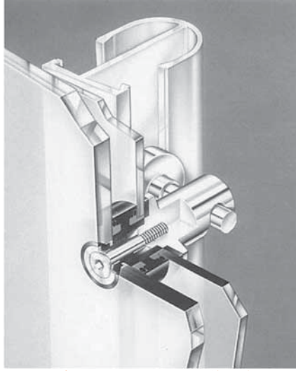
(الشكل 24.7) منظومة تزجيج مسطحة للواحيات مقدمة من بيلكينغتون.
