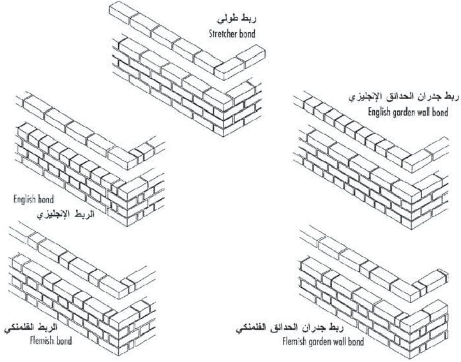
(الشكل 17.1) ربط الآجر.
