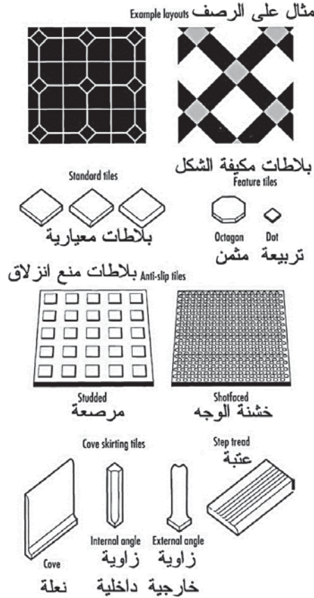
(الشكل 5.8) بلاط الأرضيات - المرقش والأملس والخاص.
