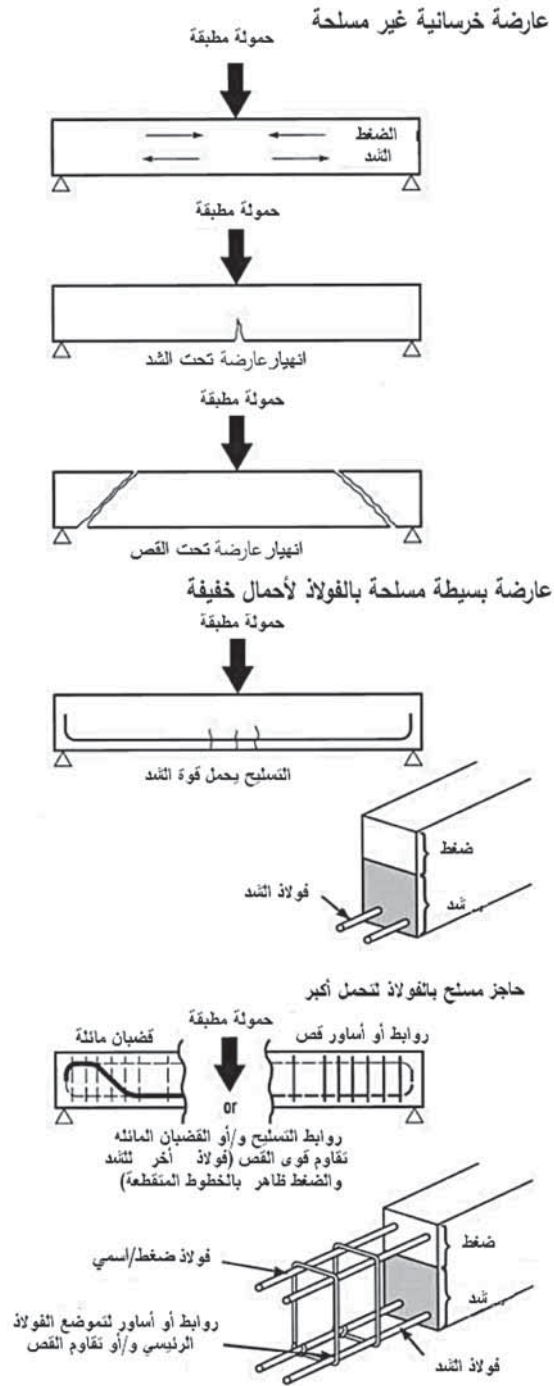
(الشكل 14.3) الخرسانة المسلحة .
