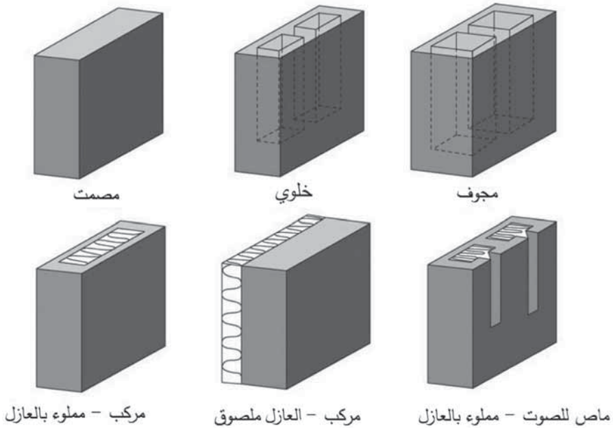
(الشكل 1.2) أنواع البلوك الخرساني.
