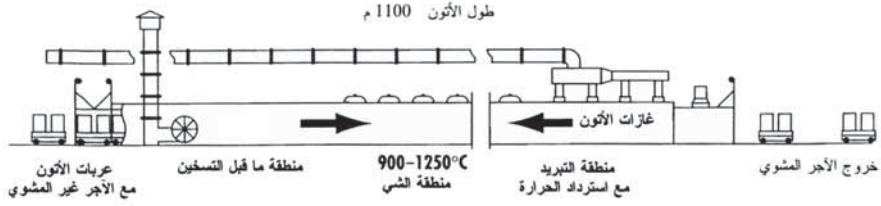
(الشكل 6.1) الفرن النفقي .
