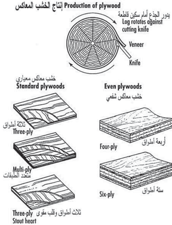
(الشكل 31.4) تصنيع وأنواع الخشب المعاكس المعياري.
