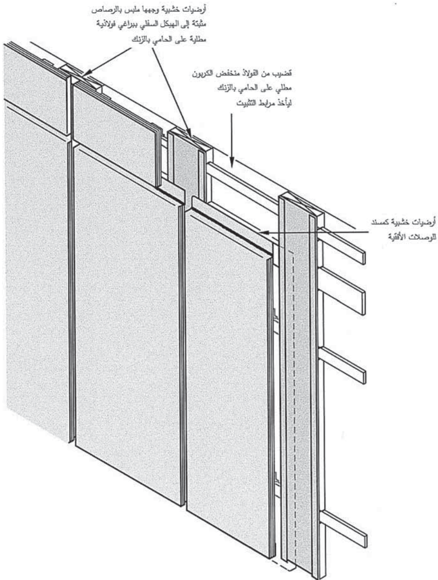
(الشكل 28.5) ألواح كسوة خشبية بوجهه من الرصاص.
