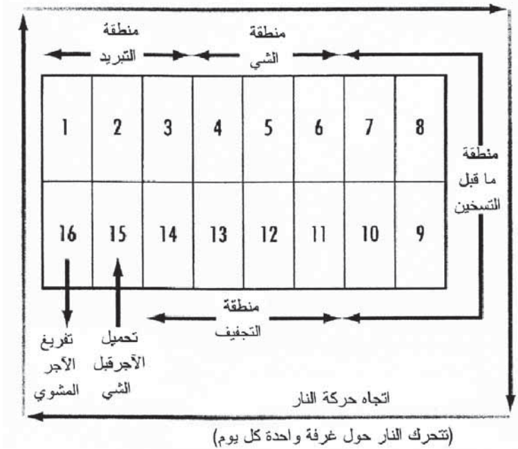
(الشكل 7.1) خطط فرن هوفمان.
