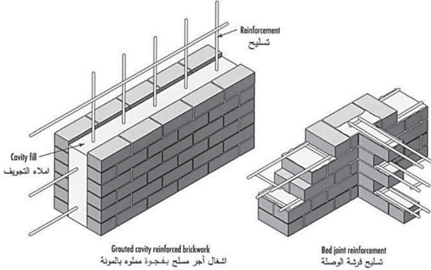
(الشكل 20.1) أشغال الآجرّ المسلح.
