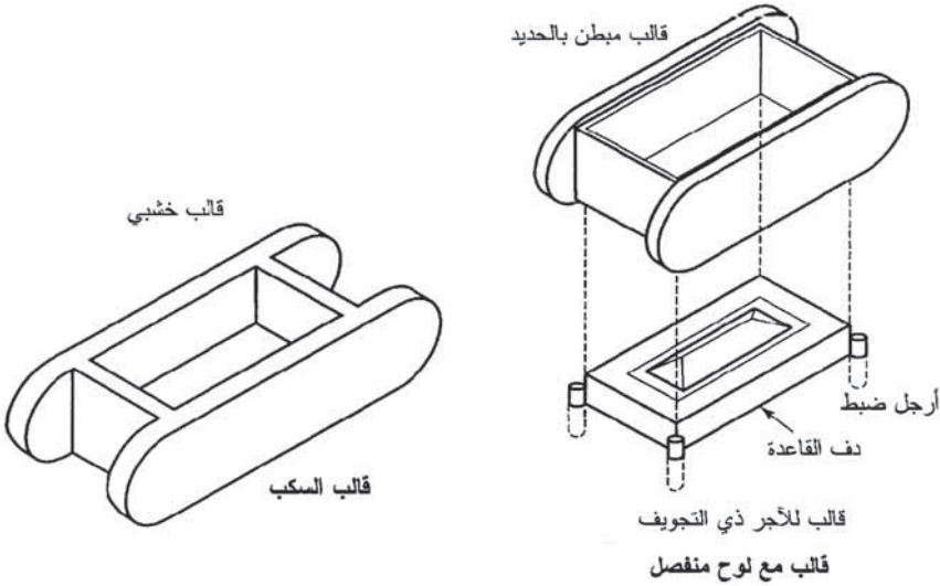
(الشكل 4.1) قوالب الآجرّ المصنّع يدوياً.
