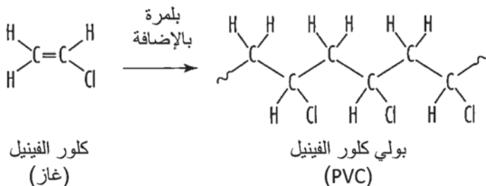
(الشكل 2.10) بلمرة كلور الفينيل إلى بولي كلور الفينيل .
