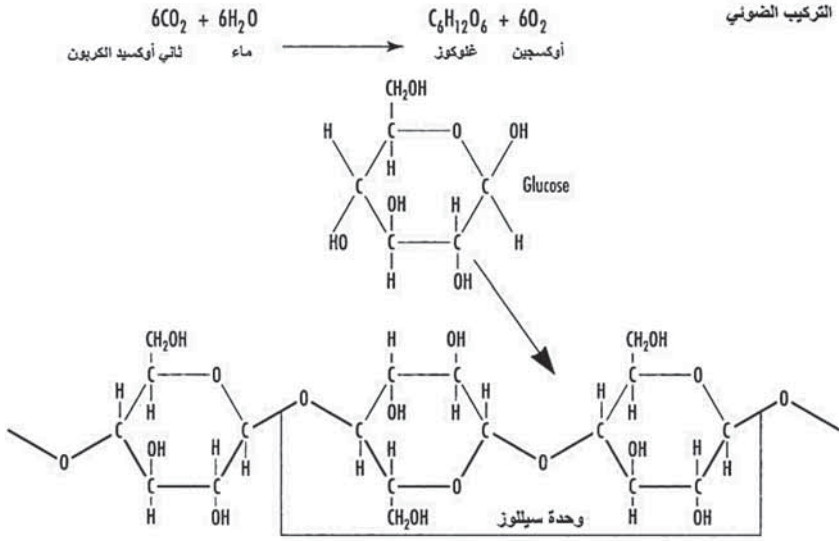
(الشكل 4.4) بنية السيلولوز.
