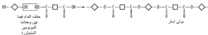
(الشكل 3.10) البلمرة بالتكاثف (Condensation polymerization) .
