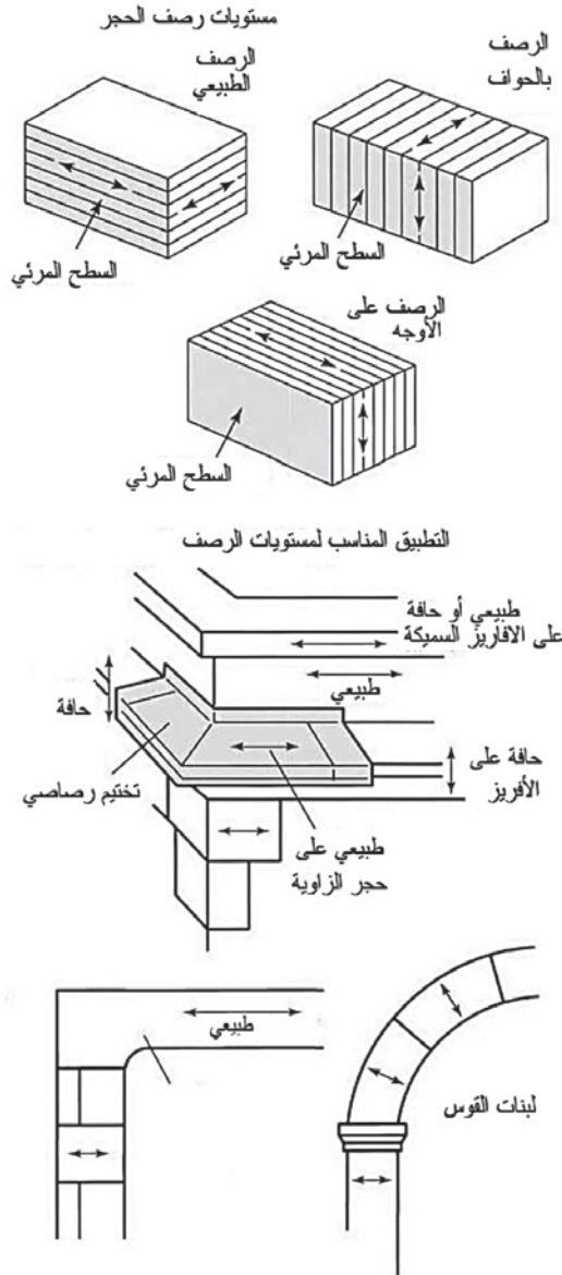
(الشكل 2.9) مستويات سرير الحجر الطبيعي.
