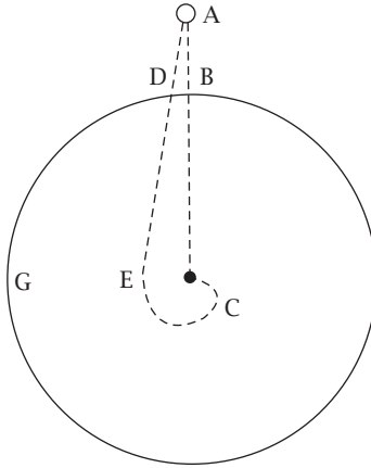
شكل ٧-١: مسار نيوتن المقترح لجسم ساقط رأسياً من أعلى سطح الأرض. ويُفترض بمسار الجسم أن يستمر إلى داخل سطح الأرض، إذ إن الأرض تدور حول نقطة المركز C عكس عقارب الساعة أي (BDG).
