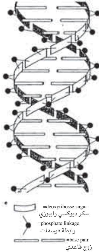
تابع شكل(2) مقطع من جزيء الحامض النووي الديوكسي رايبوزي (دنا)
