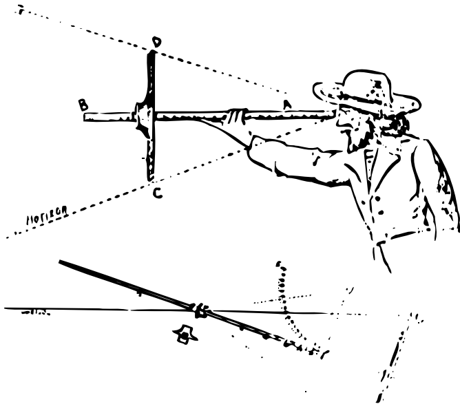
الشكل(6): آلة الارليت وتدرج العصا فيها يعتمد على نظرية الربع المجيب للخوارزمي (عن برنيسبس 1836)
