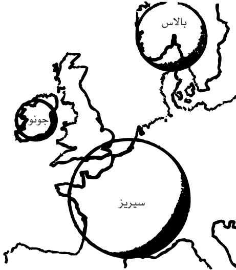
شكل (4-1): الكويكبات. حجم الكويكبات مقارناً بالبلدان الأوروبية. فسيريز وهو أكبرها يغطي مساحة فرنسا، وبالاس يغطي مساحة جنوب النرويج والسويد، وحجم جونو يقارب حجم أيرلندا.
