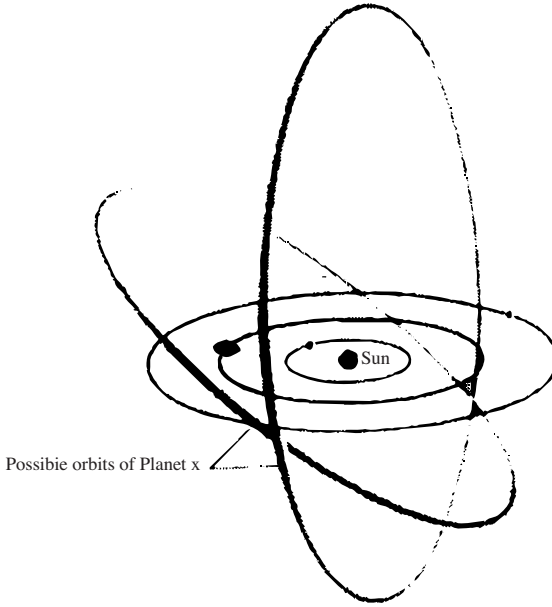
شكل (3-4). الكوكب إكس - الكوكب العاشر؟ المدارات المحتملة للكوكب إكس حسب ناسا في 1987.
