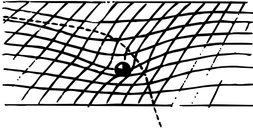
شكل (10-3) الجاذبية تسبب انبعاج المكان-الزمان. جسم ثقيل يسبب انبعاج المكان والزمان. الخط المنقطع بين المسار الذي ستتبعه كرة تتدحرج عبر هذا السطح المتخيل للمكان-الزمان. ويُفسّر الانحراف حول الانبعاج على أنه نتيجة لقوة الجاذبية.
