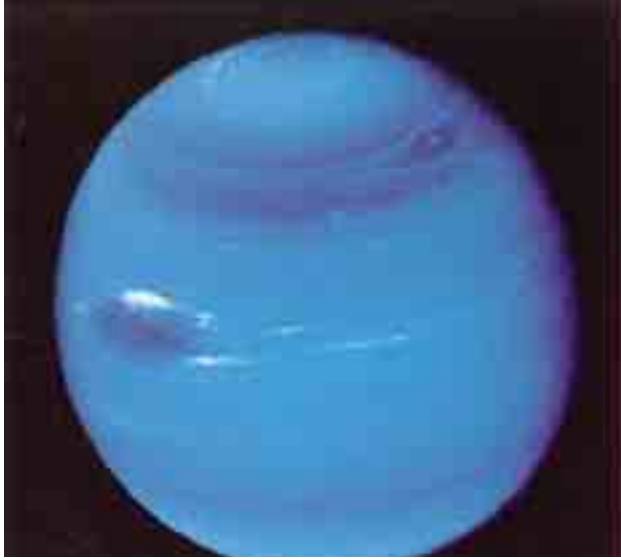
(62) صورة عن قرب لكوكب نبتون، السمات الرئيسية الثلاث للسحب، من أعلى إلى أسفل يميناً، يطلق عليها اسم «البقعة المعتمة الكبرى»، و«الدراجة»،
