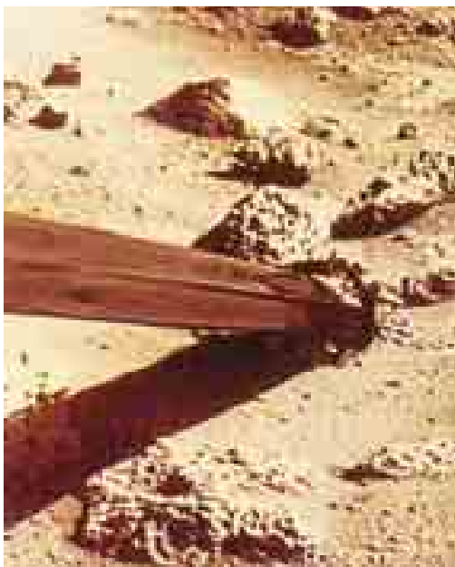
(107) تربة مريخية في ظل الأشعة فوق البنفسجية. في الصورة اليسرى، نجد ذراع جمع العينات، التابع للسفينة فايكنج، يدفع صخرة ذات بثور بعيدا عن الطريق حتى يتمكن من الحفر. وبعد الحصول على عينة التربة
