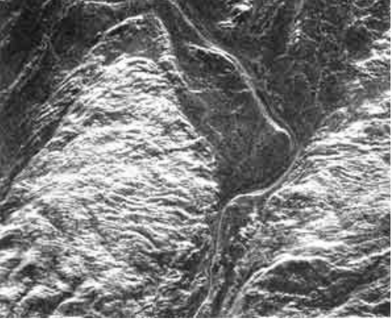
أ. قناة متعرجة شمال جبال فرويچا (Fruyja) على كوكب الزهرة، بيانات من السفينة ماجلان.
