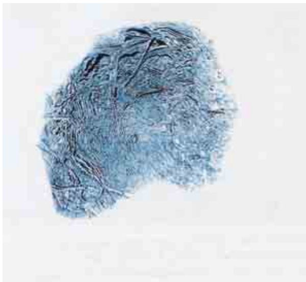
(57) أ - أرييل، قمر من أقمار أورانوس. مسقط للقطب الجنوبي.
