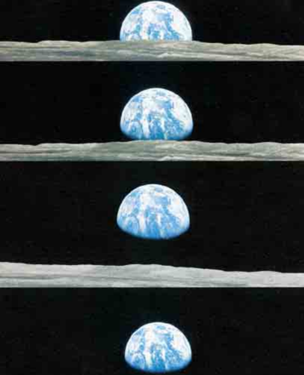
(18) تغير في المنظور: كوكب الارض يرتفع فوق حوض مارسيمي على القمر، (Mare Smythii) والناجم عن تصادم قديم، لو أننا نعيش على القمر، هل كنا سنعتبره مركز الكون. والأرض نقدم لنا فروض التبجيل؟ (صور التقطها سفينة الفضاء أبوللو . 11)
