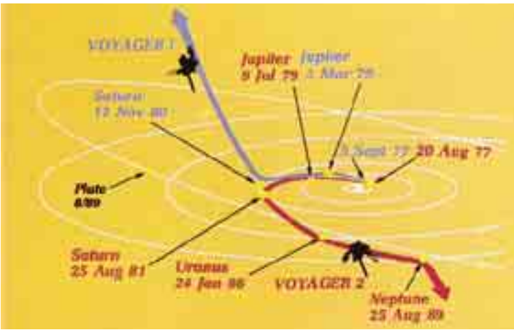
(38) أ. مسارا سفینتی الفضاء فوییجر .
