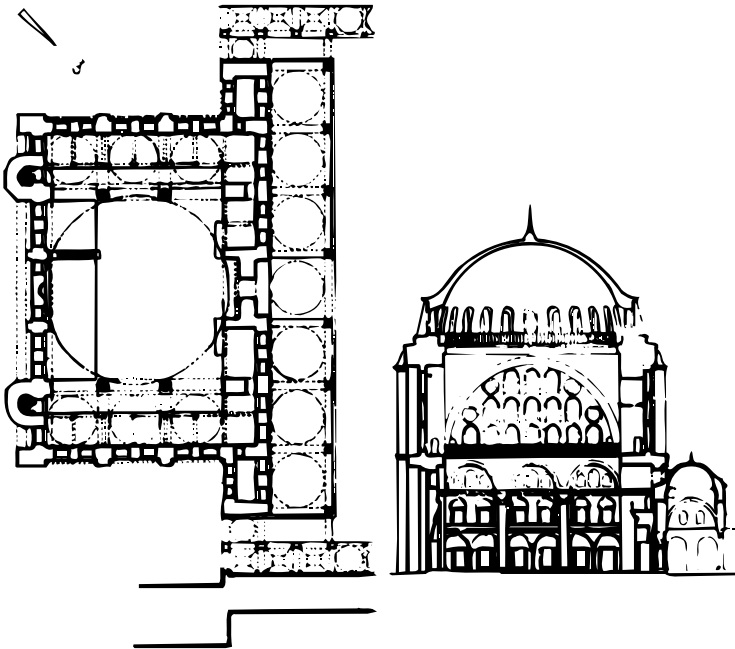
مخطط مسجد مهران في اشتابول وقطاع منه
