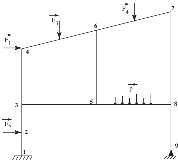
Figure 5.8 Exemple de structure hyperstatique
