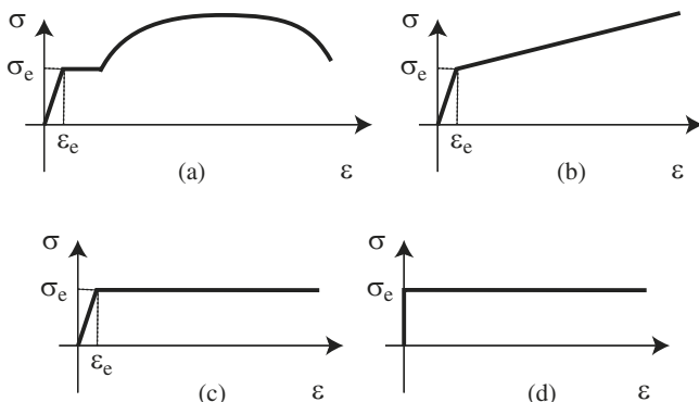
Figure 9.1 Loïs de comportement : matériau ductile (a), modèle élasto-plastique écrouissable (b), modèle élasto-plastique parfait (c), modèle rigide plastique (d)
