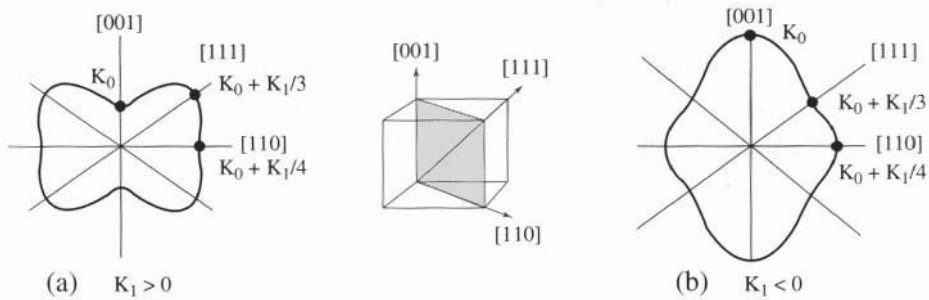
Figure 3.10 - Représentation polaire de l'énergie d'anisotropie magnétocristalline
