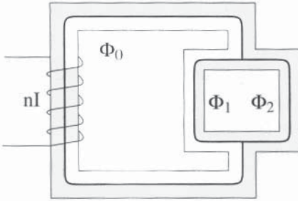
Figure 2.21 - Circuit magnétique comportant une dérivation
