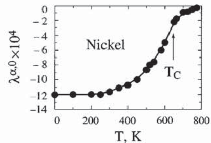
Figure 12.5 - Magnétostriction d'échange du nickel métallique [5]
