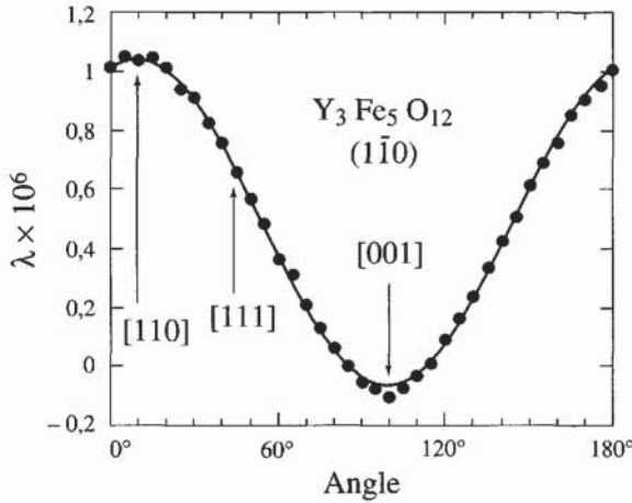
Figure 12.9 Variations azimutales de la magnétostriction d'un cristal de YIG mesurée selon [1-10] lorsque le champ magnétique tourne dans le plan perpen- diculaire à cette direction
