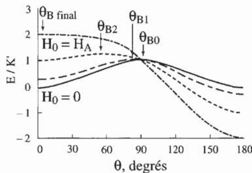
Figure 5.52 - Évolution de la barrière d'énergie avec le champ appliqué
