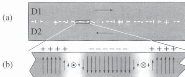
Figure 5.13 - Parois observées par méthode de Bitter sur une couche mince de Fe-Ni de 100 nm d'épaisseur, d'après [6]
