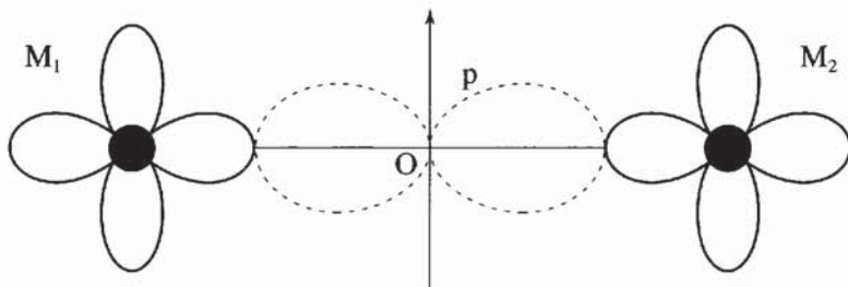
Figure 9.1 - M_1 et M_2 : ions de transition, O : ion O^{2-}
