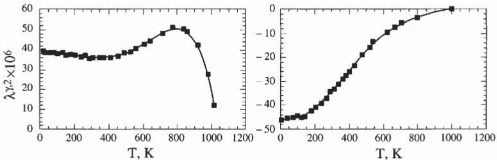
Figure 12.11 - Variations thermiques des coefficients de magnétostriction d'un monocristal de fer : à gauche, mesure selon la direction [100] ; à droite, mesure selon la direction [111], d'après [10]
