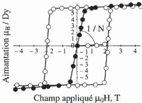
Figure 5.36 - Cycles d'hystérésis du composé Dy_3Al_2 à 4,2 K (o) et à 30 K (•) [4]
