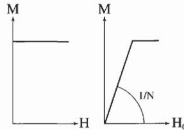
Figure 2.18 - Courbes d'aimantation schématisées en fonction du champ interne ( H ) et du champ externe ( H_0 ) pour une substance présentant une susceptibilité infinie
