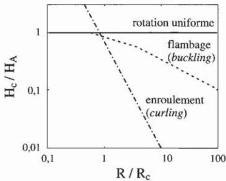
Figure 5.59 - Comparaison des champs de retournement selon différents processus en fonction du diamètre de grain dans le cas d'un matériau sans anisotropie magnétocristalline
