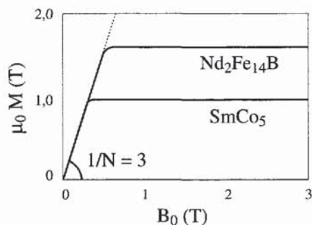
Figure 5.31 - Courbes d'aimantation des composés \text{SmCo}_5 et \text{Nd}_2\text{Fe}_{14}\text{B} taillés sous forme de sphères
