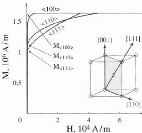
Figure 3.15 - Courbes d'aimantation d'un monocristal de fer (symétrie cubique) lorsque le champ est appliqué selon les trois directions de haute symétrie
