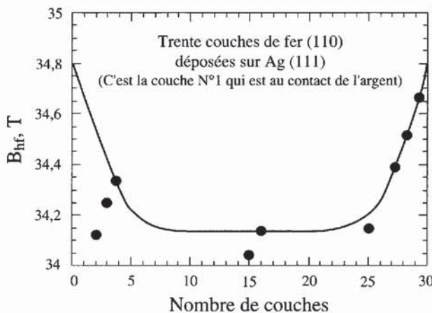
Figure 8.11 - Variations du champ hyperfin en fonction de la position de la sonde Fe^{57} dans des films de 30 couches de Fe (110) déposées sur Ag (111) à 4.2 K [8].
