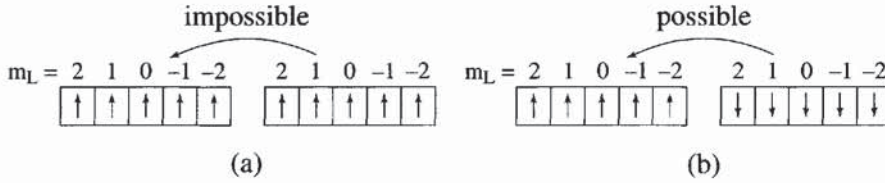
Figure 9.7 - Antiferromagnétisme d'une bande à moitié pleine
