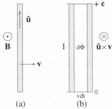
Figure 2.23 - Conducteur (a) en mouvement (b)
