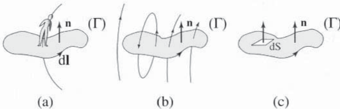
Figure 2.2 - Théorème d'Ampère
