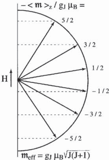
Figure 4.8 - Quantification du moment magnétique ( J = 5/2 )
