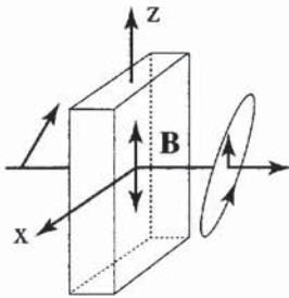
Figure 13.3 - La biréfringence quadratique due à un champ ou une aimantation suivant z entraîne un déphasage entre les composantes de \mathbf{E} suivant x et suivant z
