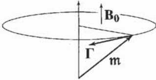
Figure 4.4 - Précession d'un moment magnétique \mathbf{m} autour d'un champ d'induction magnétique \mathbf{B}
