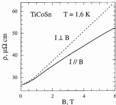
Figure 14.4 - Magnétorésistance de type cyclotron pour B/I et B⊥I
