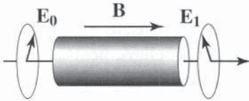
Figure 13.1 Géométrie de l'effet Faraday
