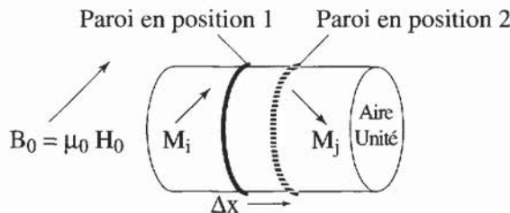
Figure 5.34 - Pression exercée sur une paroi, après application de B_0 // M_i
