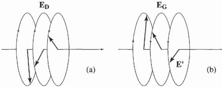
Figure 13.10 - Vibrations circulaires droite (a) et gauche (b)
