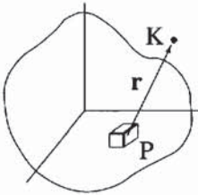
Figure 2.27 - Le point K est hors de la matière magnétique
