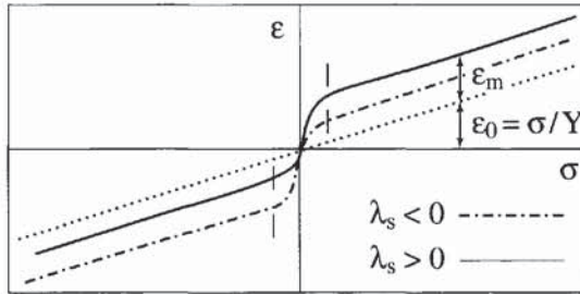
Figure 12.31 - Courbe déformation-contrainte pour un ferromagnétique
