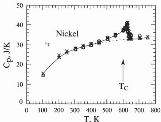
Figure 11.1 - Variations thermiques de la capacité calorifique molaire du nickel, d'après Ahrens ( \Delta ), Grew (o) et Lapp ( \times ) [1]
