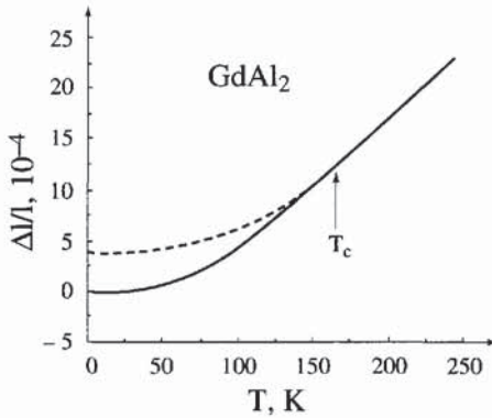
Figure 3.19 - Dilatation thermique longitudinale du composé \text{GdAl}_2 [10]
