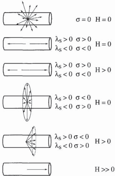
Figure 12.27 - Comportement sous contrainte uniaxiale des substances ferromagnétiques : apparition d'une anisotropie induite
