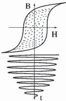
Figure 6.24 - Désaimantation sous champ alternatif évanescent
