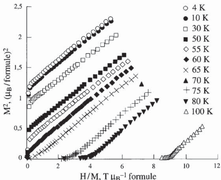
Figure 4.25 - Tracés d'Arrott pour un très faible ferromagnétique, \text{Lu}_3\text{C}_{07,77}\text{Sn}_4 [8]
