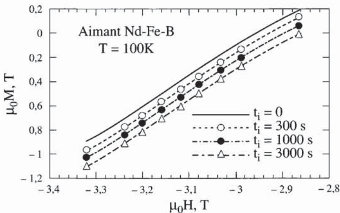
Figure 6.35 - Portions de la même zone du cycle d'hystérésis proches du champ coercitif d'un aimant Nd-Fe-B, obtenues point par point à 100 K, après avoir attendu un temps t_i variable. La courbe en trait plein, inaccessible à l'expérience, est déduite des autres grâce à la relation (6.51).
