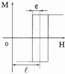
Figure 6.26 – Cycle élémentaire de Preisach
