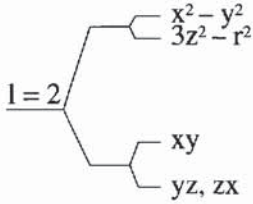
Figure 8.8 Pérovskites à base de cuivre
