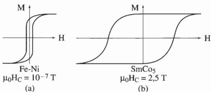
Figure 6.29 - Cycles d'hystérésis du Fe-Ni (doux) et du SmCo 5 (dur)
