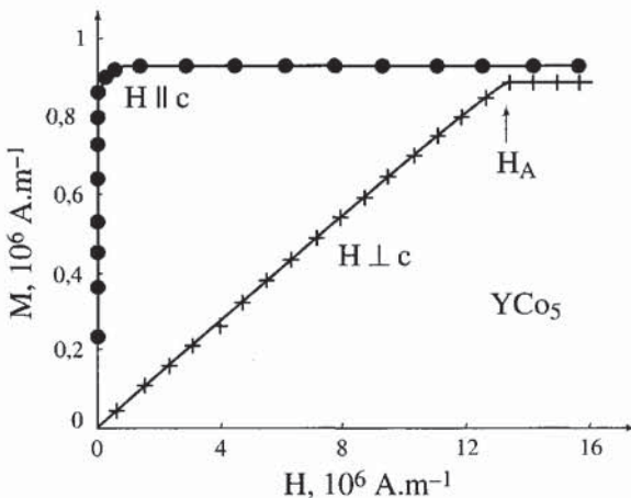
Figure 3.13 - Variations de l'aimantation en fonction du champ interne mesurées à 4,2 K sur un monocristal du composé hexagonal YCo_5 , d'après [3]
