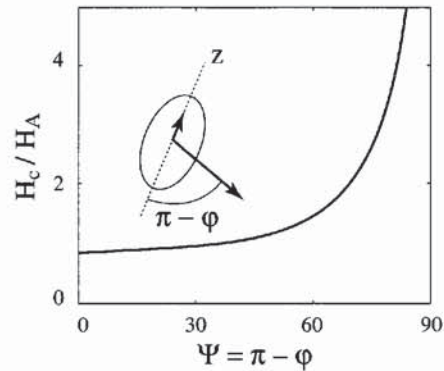
Figure 5.60 - Dépendance angulaire calculée du champ de renversement irréversible H_c , lorsque le renversement n'est précédé par aucune rotation réversible des moments (loi en 1/\cos \theta_H )
