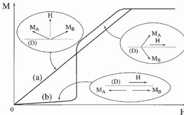
Figure 4.15 - Représentation schématique du processus d'aimantation à basse température d'un matériau antiferromagnétique à faible anisotropie magnétocristalline (a) H \perp (D) - (b) H \parallel (D) : dans ce dernier cas, on observe une transition métamagnétique
