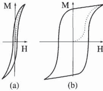
Figure 6.30 - Processus dominant : piégeage de parois
