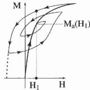
Figure 6.25 - Courbe d'aimantation anhystérétique
