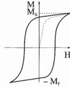
Figure 6.31 - Processus dominant : nucléation
