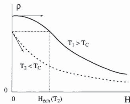
Figure 14.6 - Magnétorésistance en fonction du champ dans le domaine para- ou ferromagnétique
