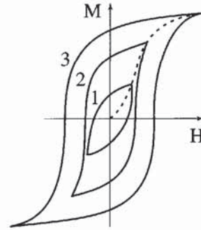
Figure 6.20 - Cycles mineurs et majeur
