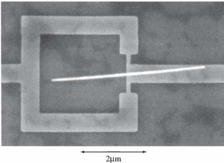
Figure 1.9 - Microsquid réalisé au L2M - CNRS, Bagnex par D. Mailly
