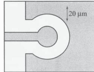
Figure 1.5 - Microbobine créant un champ magnétique de 40 teslas
