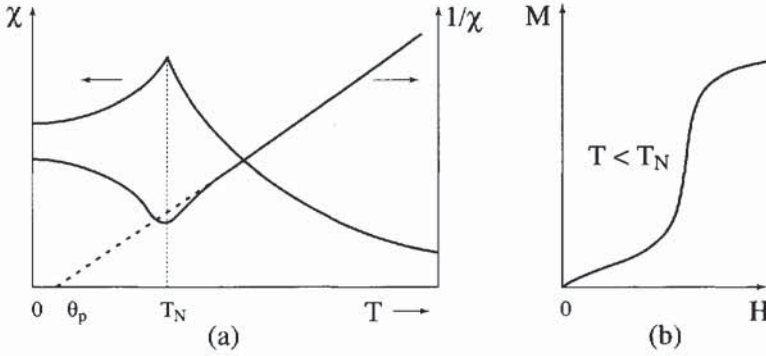
Figure 4.13 - (a) Représentation schématique des variations expérimentales de la susceptibilité et de son inverse pour un matériau antiferromagnétique (b) Allure de l'aimantation en fonction du champ, en dessous de la température d'ordre T_N
