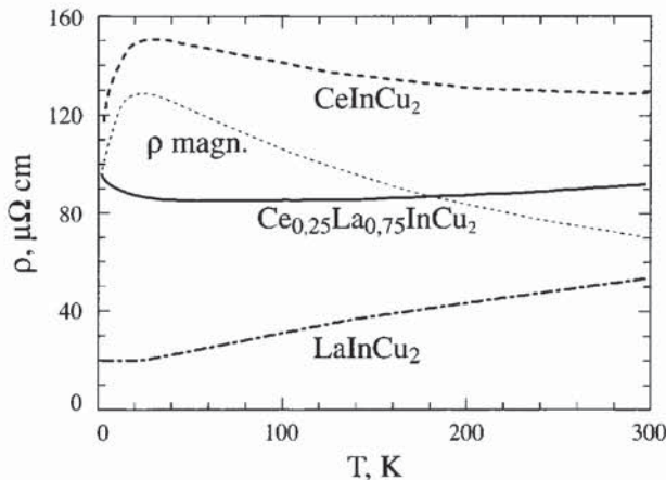
Figure 14.3 - Résistivité des composés \text{CeInCu}_2 (Kondo), \text{LaInCu}_2 (non magnétique) et d'une solution solide (\text{Ce},\text{La})\text{InCu}_2
