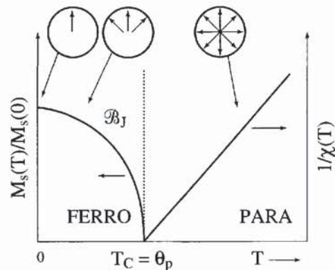
Figure 4.11 - Représentation théorique de la variation thermique de M_s et de \chi^{-1} paramagnétique dans un ferromagnétique simple
