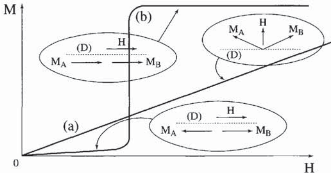
Figure 4.16 - Représentation schématique du processus d'aimantation à basse température d'un matériau antiferromagnétique à forte anisotropie magnétocristalline (a) H \perp (D) - (b) H \parallel (D) : dans ce dernier cas, on observe une transition métamagnétique
