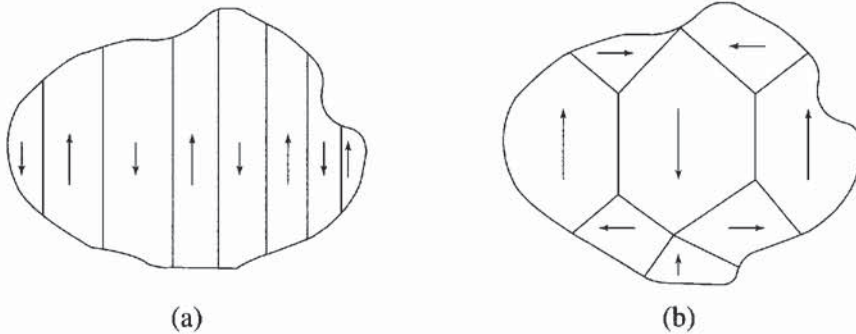
Figure 3.9 - Représentation schématique de la division en domaines (a) Cristal hexagonal où l'axe sénaire [001] est de facile aimantation (b) Cristal cubique où les axes quaternaires \langle 100 \rangle sont de facile aimantation (la notation \langle 100 \rangle désigne l'ensemble des directions [100], [010] et [001])
