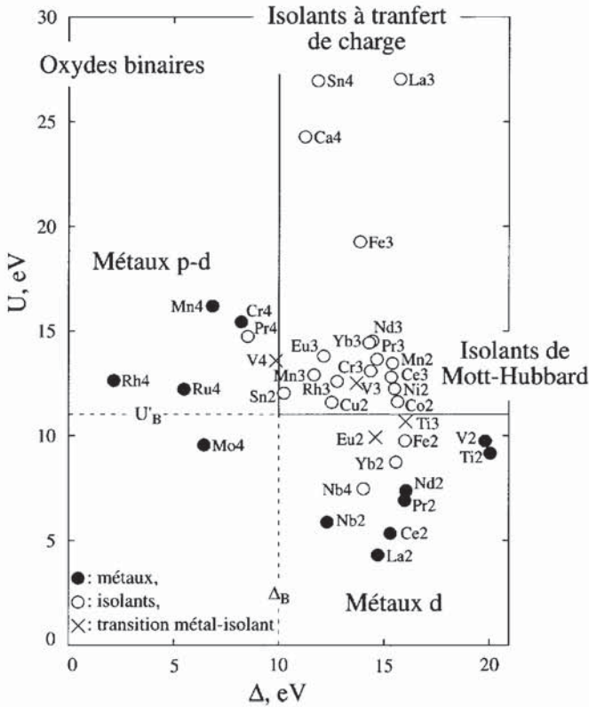
Figure 14.8 - Classification de 38 oxydes binaires, d'après [27] Nomenclature selon Zaanen, Sawatzky, Allen [26]
