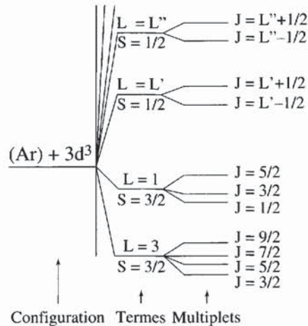
Figure 7.7 - Décomposition de la configuration fondamentale de l'ion Cr^{3+} en termes et en multiplets
