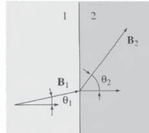
Figure 2.19 Le dioptre magnétique
