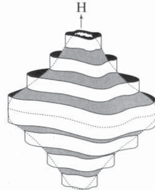
Figure 14.10 - Quantification des aires des orbites (Ziman)
