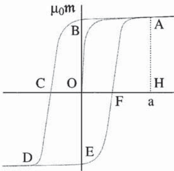
Figure 11.5 Cycle d'hystérésis
