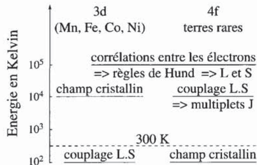
Figure 7.10 – Ordre de grandeur des différentes interactions agissant sur les atomes 3d et 4f dans la matière
