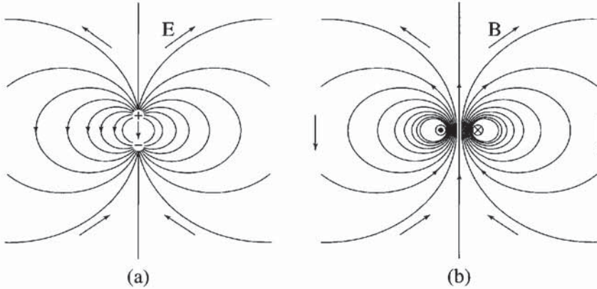
Figure 2.7 - (a) Champ électrique engendré par une paire de charges égales et opposées (b) Induction magnétique engendrée par une boucle de courant
