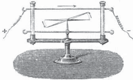
Figure 1.3 - L'expérience historique d'Ersted d'après [7]
