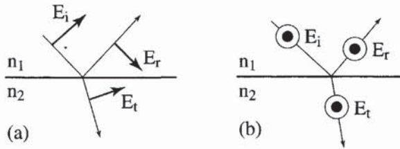
Figure 13.11 - Réfraction et réflexion à un dioptre plan : (a) Polarisation p ou TM - (b) Polarisation s ou TE
