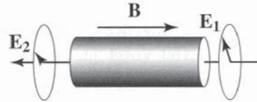
Figure 13.2 Caractère non-réciproque de l'effet Faraday
