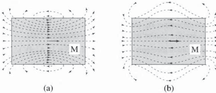
Figure 2.13 - Lignes de champ (a) de l'induction \mathbf{B} et (b) du champ \mathbf{H} , en présence d'un cylindre uniformément aimanté. En tout point du matériau, \mathbf{H} = (\mathbf{B}/\mu_0) - \mathbf{M} .
