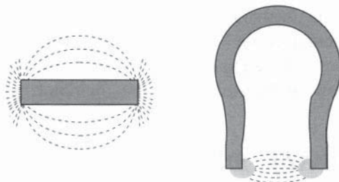
Figure 1.2 - Le spectre magnétique d'un aimant
