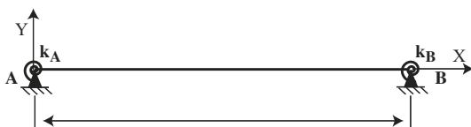
Figure 5.20 Poutre à une travée avec des encastres élastiques à ces extrémités
