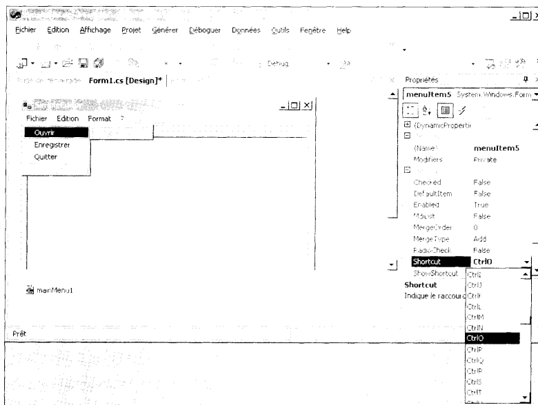
Figure 17.6 : La propriété Shortcut permet de spécifier le raccourci clavier que vous voulez assigner à l'élément de menu.
