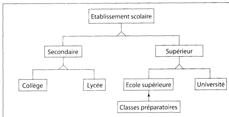
Figure 13.4 : Le factoring produit généralement des couches supplémentaires dans la hiérarchie d'héritage.
