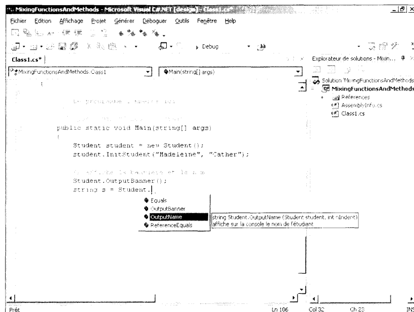
Figure 8.6 : Avec un programme documenté en XML, Visual Studio est capable de bien mieux décrire la fonction et ses arguments.
