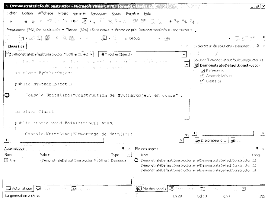
Figure 11.3 : Le contrôle passe dans le construc- teur
