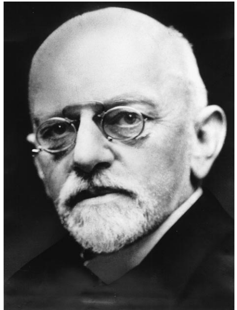
David Hilbert (1862-1943) était, avec le Français Henri Poincaré, l'un des grands mathématiciens des années 1900. Par la profondeur de ses travaux et de ses points de vue, par le dynamisme qu'il a su insuffler à Göttingen, il a exercé une influence considérable sur les mathématiques du XX e siècle. (Cliché AKG)
