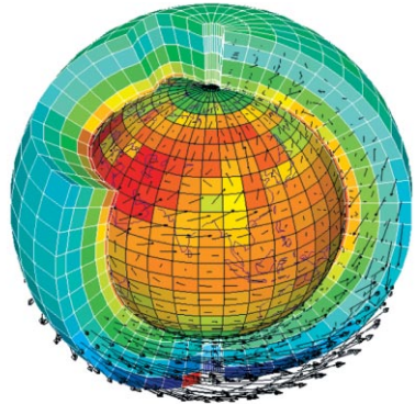
Vue d'artiste des boîtes de calcul d'un modèle de prévision du temps ou du climat. (Illustration L. Fairhead LMD/CNRS).
