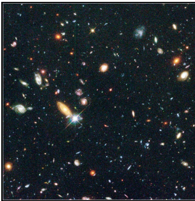
Une myriade de galaxies très lointaines vues par le télescope spatial Hubble. La gravitation étant un élément clef de la naissance et de l'évolution de l'Univers, les spécialistes de cosmologie aimeraient disposer enfin d'une description de la force de gravitation compatible avec les principes de la physique quantique. La théorie des cordes exaucera-t-elle ce vœu ? (Cliché R. Williams/HDF (STSci)/NASA)
