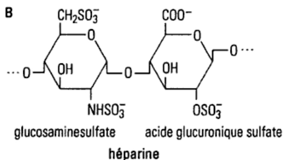
Fig. 3 – Exemples d'hétérosides.
