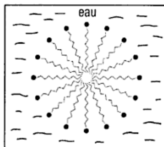
Fig. 5 – Micelle.
