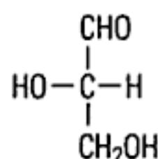
L-glycéraldéhyde
