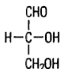
D-glycéraldéhyde
