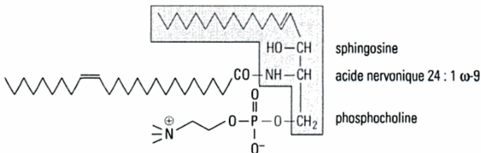
Fig. 3 – Une sphingomyéline.
