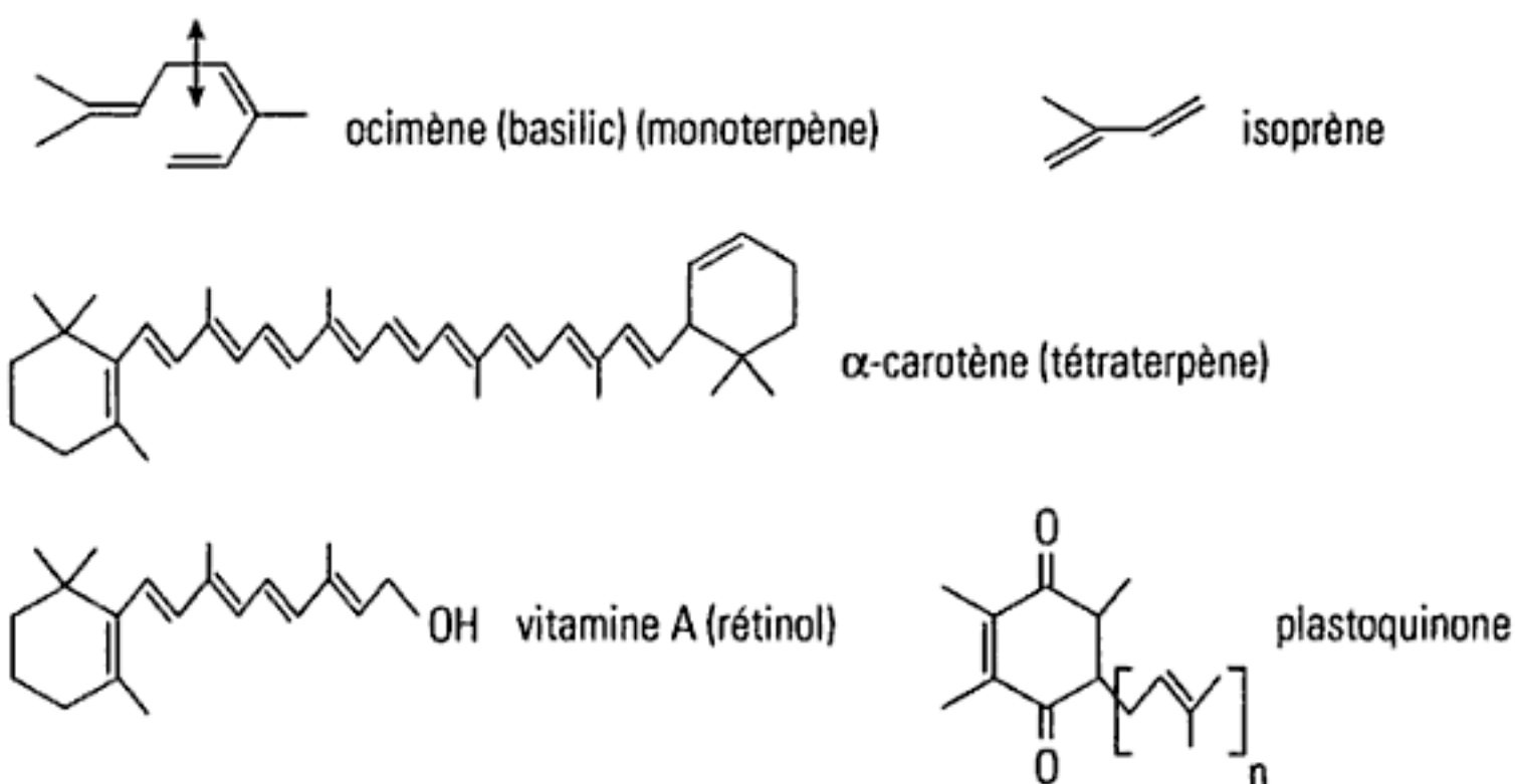
Fig. 6 – Isoprénoïdes.
