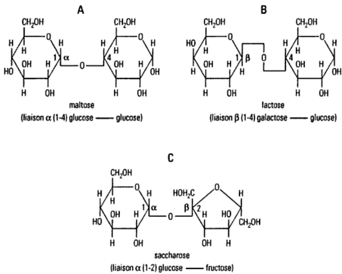
Fig. 1 – Principaux diholosides.
