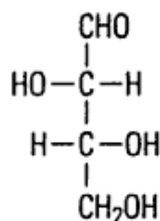
D-thréose
