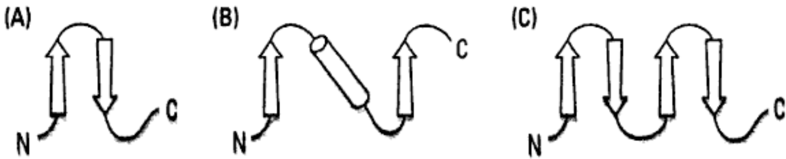
Fig. 5 – Structures super-secondaires ou motifs : (A) Structure \beta - \beta ou motif en épingle à cheveux (2 feuillets \beta antiparallèles) (B) Structure \beta - \alpha - \beta (2 feuillets \beta parallèles, une hélice \alpha ) (C) Disposition de 4 feuillets \beta antiparallèles
