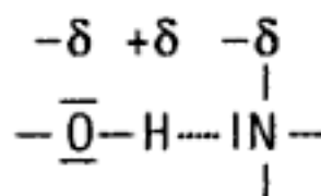
Fig. 3 – Liaison hydrogène.
