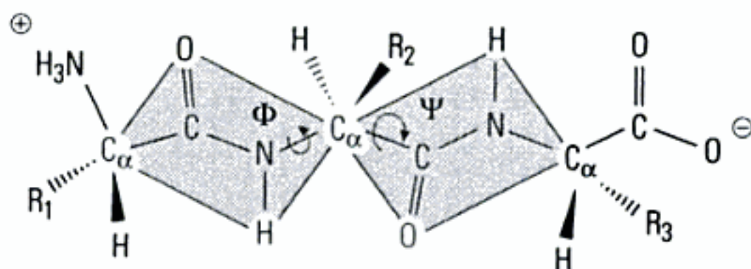
Fig. 1 – Chaîne peptidique – Les deux angles \Phi (autour de la liaison C_\alpha-N ) et \Psi (autour de la liaison C_\alpha-C ) définissent les positions relatives des plans des deux liaisons peptidiques. Les rotations sont limitées par l'encombrement stérique.
