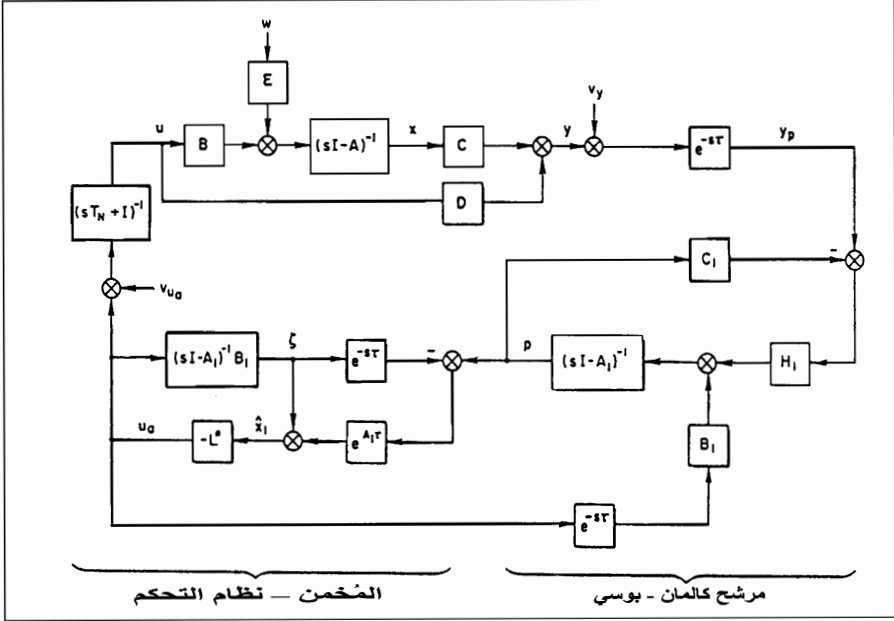
الشكل 21 - 2 نموذج الطيار الحسائي، المستخدم في حلقة التحكم الأمثل. تتضمن مصفوفات الطائرة A, B, C, D مرشح تشكيل الضجيج E، في الجزء العلوي اليساري. يتم التنبؤ عن حالات الطائرة بواسطة مرشح كالمان - بوسي (Kalman - Bucy) في الجزء الأيمن السفلي. ويقع نظام التحكم الأمثل في الجزء السفلي الأيسر. (من: Thompson, AIAA Paper 88- (4183, 1988).
