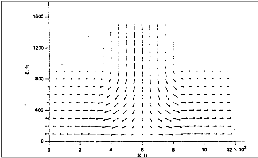
الشكل 18 - 11 المقطع العمودي العرضي في نموذج برنه للدفق السفلي (Bray model of down - burst). طول الأسهم متناسبة مع سرعة جريان الهواء (من : Bray, NASA TM 85969, 1984).
