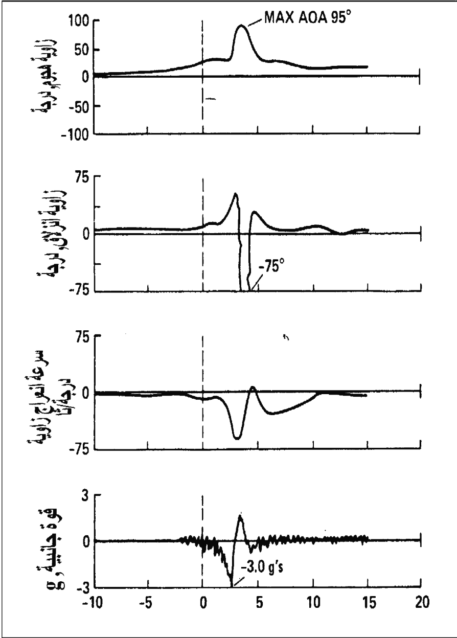
الشكل 9 - 13 مغادرة الانعراج على الحدود الصوتية التي تم الحصول عليها مع الطائرة ماك دونيل دوغلاس F/A-18A باستخدام التحكمات ما قبل الحركة الحلزونية، أو دفات درجة ودفة اتجاه مضادة، مع الدرحة بزواوية هجوم وسطية (من: Anderson, Enevoldson, and Nguyen, AGARD CP-347, 1983).
