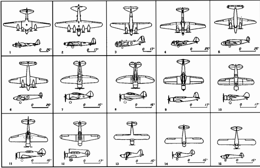
الشكل 3 - 7 الطائرات الخمسة عشرة التي اختبرها جيلروث ووايت لتزويد طريقة لتوفير معلومات عن استقرارها الطولي (من تقرير NACA رقم 711، 1941).
