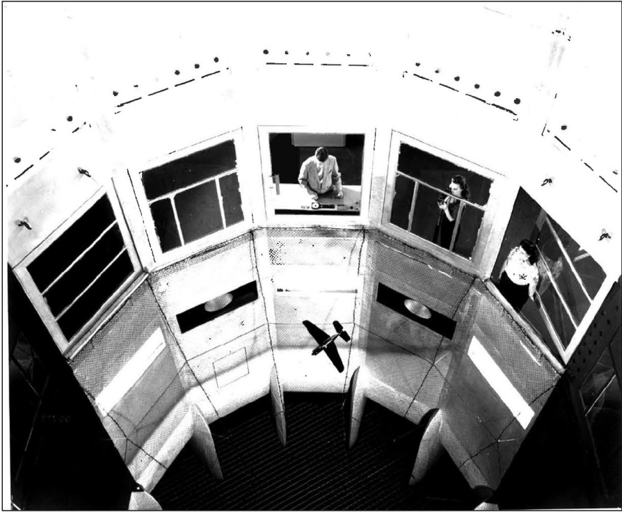
الشكل 9-2 نموذج طائرة ينهار حلزونياً في قسم اختبار الانهيار الحلزوني الحر في النفق الهوائي الذي يبلغ ارتفاعه 20 قدماً والموجود في وكالة الناسا (من : Neihouse, Kliner, and Scher, NASA Rept. R-57, 1960).
