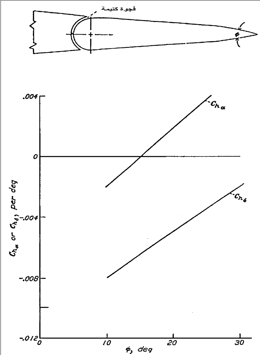
الشكل 5-8 تغيير معيار عزم المفصل المثالي مع زاوية الشد \phi لسطح تحكم مشدوف. (من: Phillips, NACA Rep. 927, 1948).
