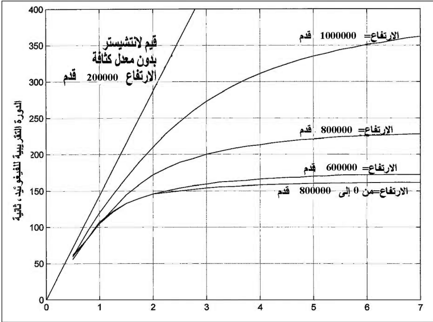
الشكل 11 - 17 تغيرات تقرب دور الحركة الاهتزازية البطيئة (الفيغويد) مع الارتفاع ورقم ماخ، متضمنة معدل الكثافة مع تأثيرات الارتفاع.
