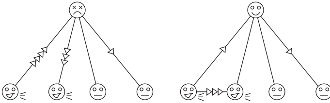
شكل ٩-٣: خوارزمية مثالية محليًا. يتم تجاوز نقطة التلاقي الأكثر ازدحامًا عن طريق إضافة رابط بين النقطتين المتجاورتين اللتين يُرسل إليهما معظم الرسائل (المشار إليهما بالأشهر).
