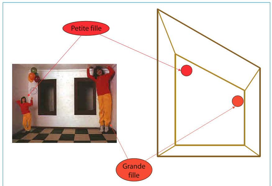
Figure 3.37 – Dans la célèbre chambre de Ames, on a l'illusion d'un petit personnage... tout en ayant l'impression se faire avoir !
