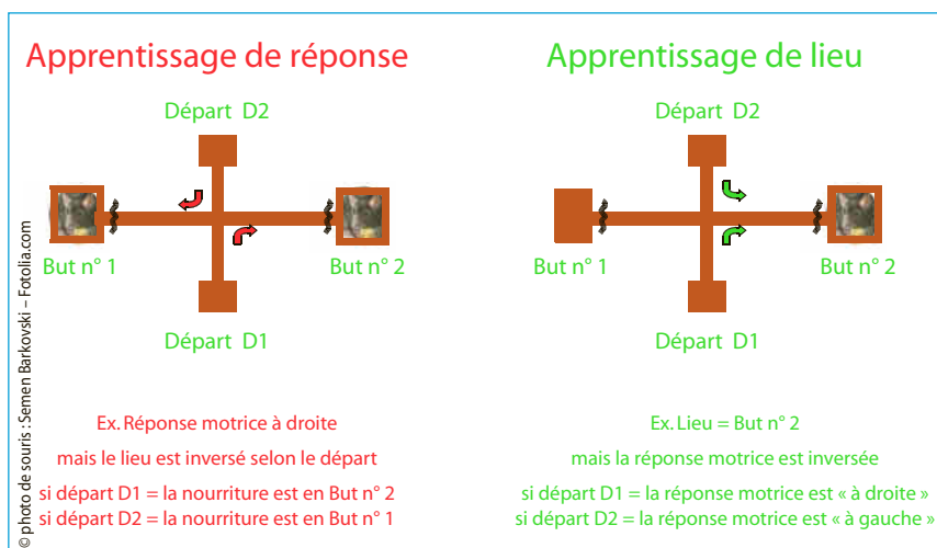
Figure 4.19 – Comparaison entre l'apprentissage de réponse et l'apprentissage de lieu.
