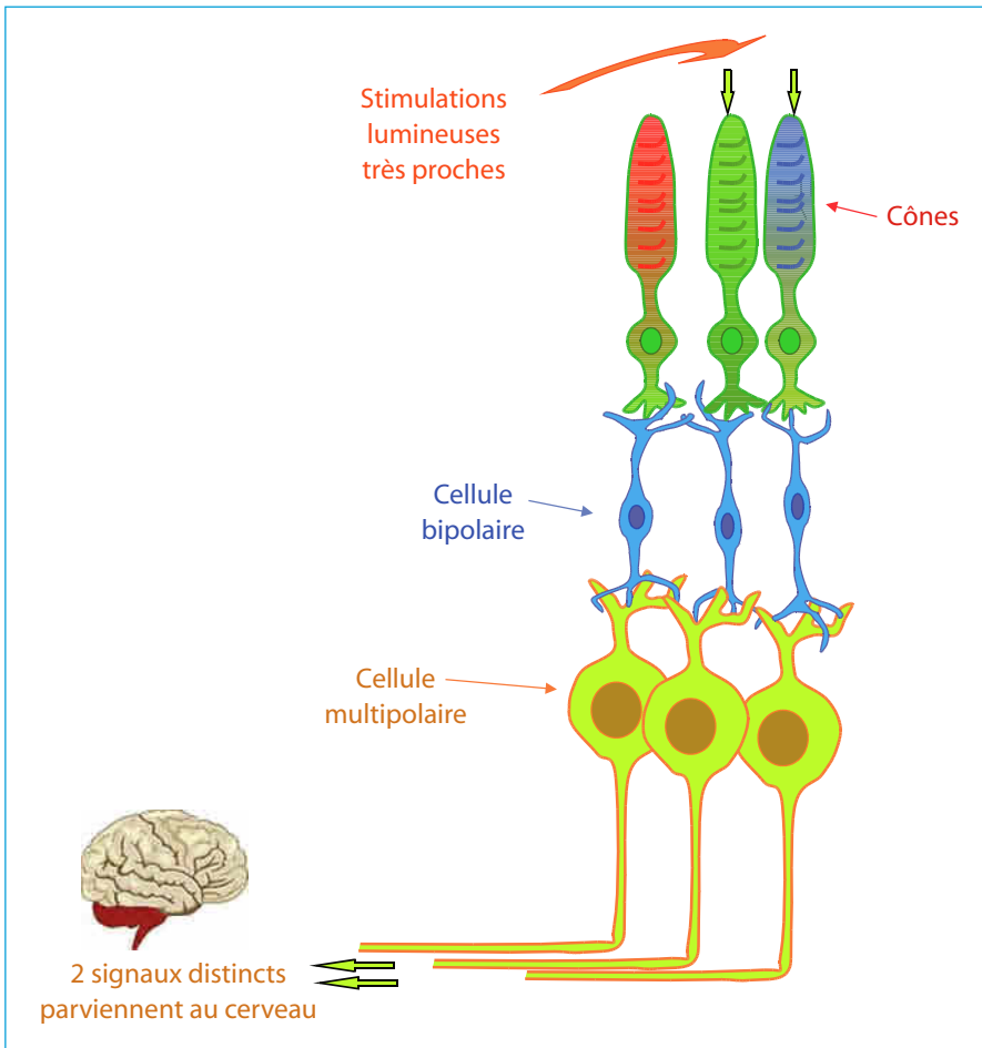
Figure 3.16 – Câblage direct en fovéa.
