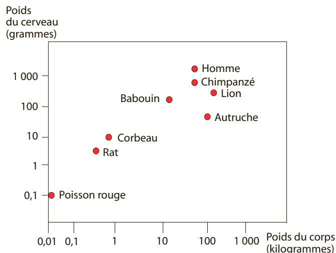
Figure 8.25 – Comparaison du poids du cerveau par rapport au poids du corps chez différents vertébrés (simplifié d'après Jerison, 1973 ; cit. Eccles, 1981).
