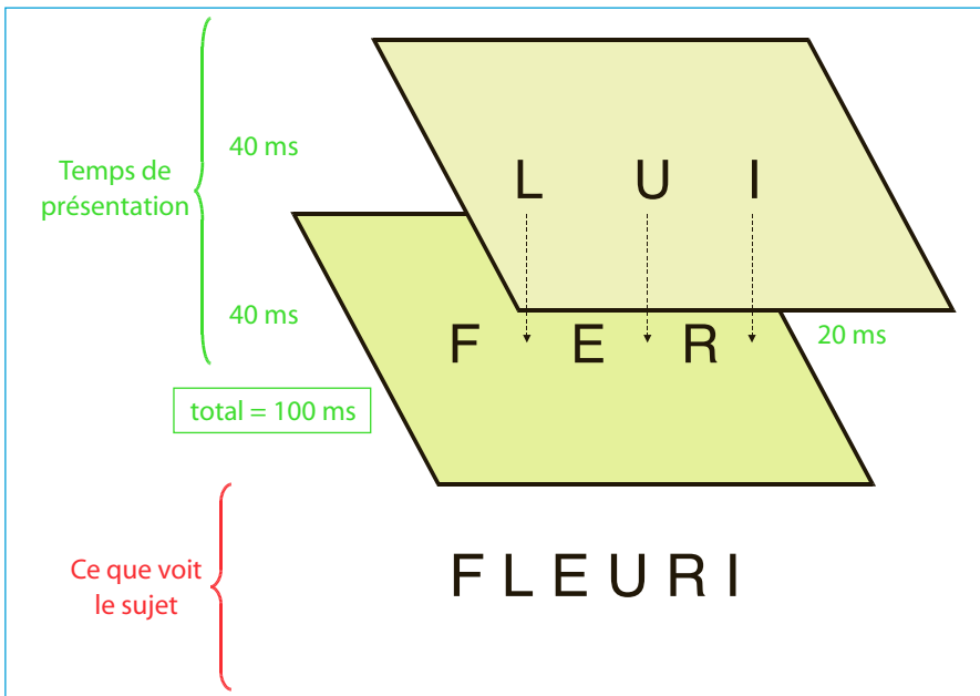
Figure 3.34 – Expérience montrant la fusion temporelle en deçà de 100 ms (d'après Fraisse, 1968).
