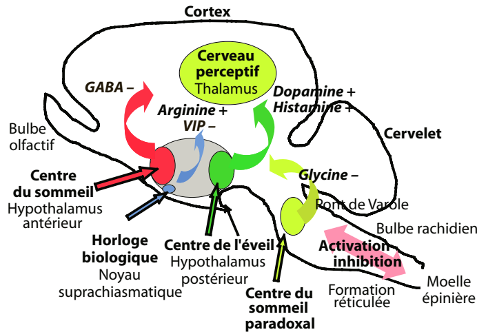
Figure 6.3 – Circuits de l'éveil et du sommeil avec leurs centres et leurs neurotransmetteurs chez le chat (simplifié d'après Jouvet, Valatx, 1998).
