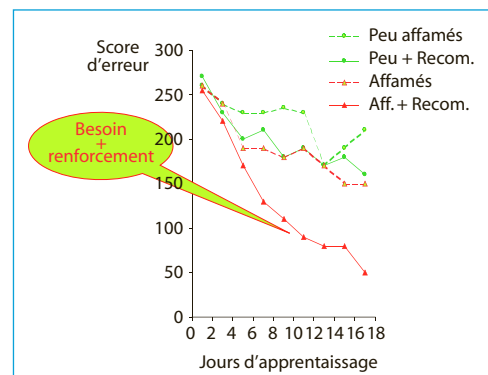
Figure 9.3 – Double effet du besoin et de la récompense chez le rat dans un labyrinthe (simplifié d'après Tolman et Honzik, 1930).
