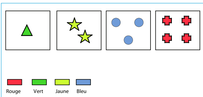
Figure 6.10 – Test de classement de cartes du Wisconsin d'après Milner (cit. Shallice, 1995).
