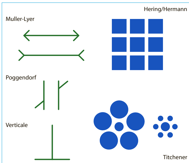
Figure 3.32 – Exemples d'illusions : d'assimilation (à gauche) et de contraste (à droite).
