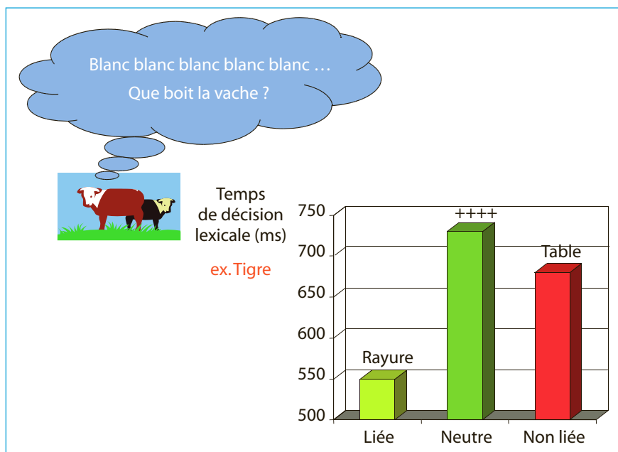
Figure 5.20 – Amorçage dans la décision lexicale.
