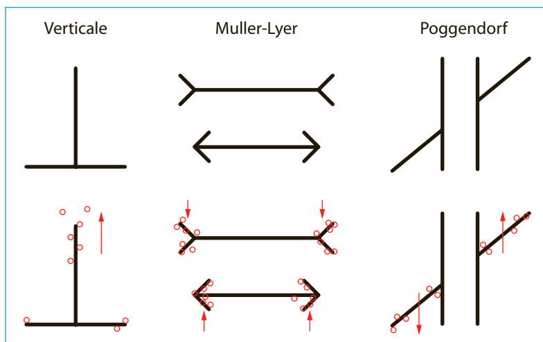
Figure 3.33 – Explication des illusions d'assimilation en termes de densité de fixations.
