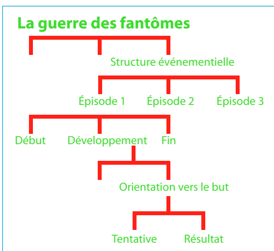
Figure 7.5 – Structure hiérarchique du récit La Guerre des fantômes (simplifié d'après Mandler et Johnson, 1977).
