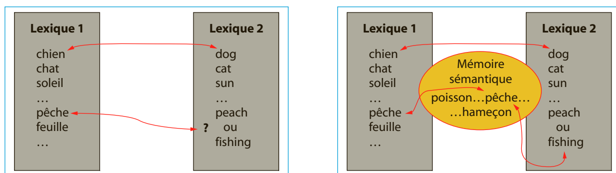
Figure 5.17 – Modèle de Quillian (1969).
