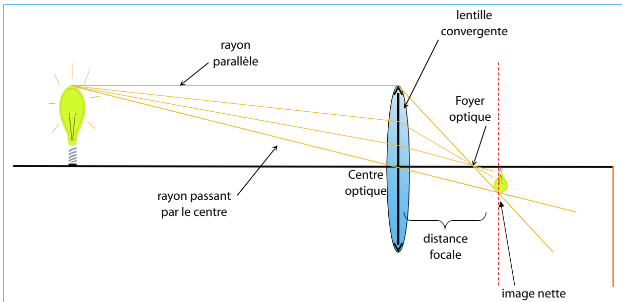
Figure 3.2 – La formation d’une image à travers une lentille convergente et dans l’œil. L’image est renversée sur l’écran (ou sur le fond de l’œil). Remarque : en optique, une lentille convergente est symbolisée par des flèches vers l’intérieur.
