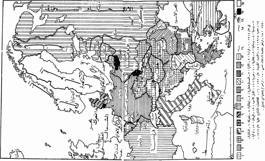
شكل ١ - تقسيم الجبهة والقطاعات القتالية عقب الحرب العالمية الأولى.
