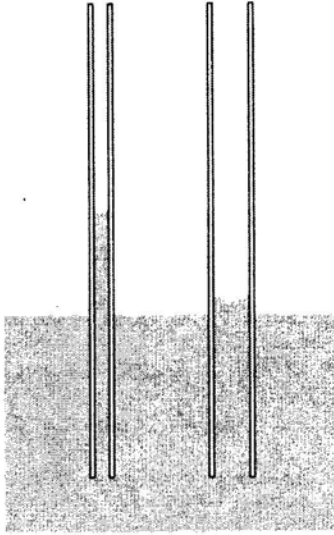
مستوى الزئبق أقل في الأنبوبة الضيقة. وينحني السطح الهلالي لأعلى.
