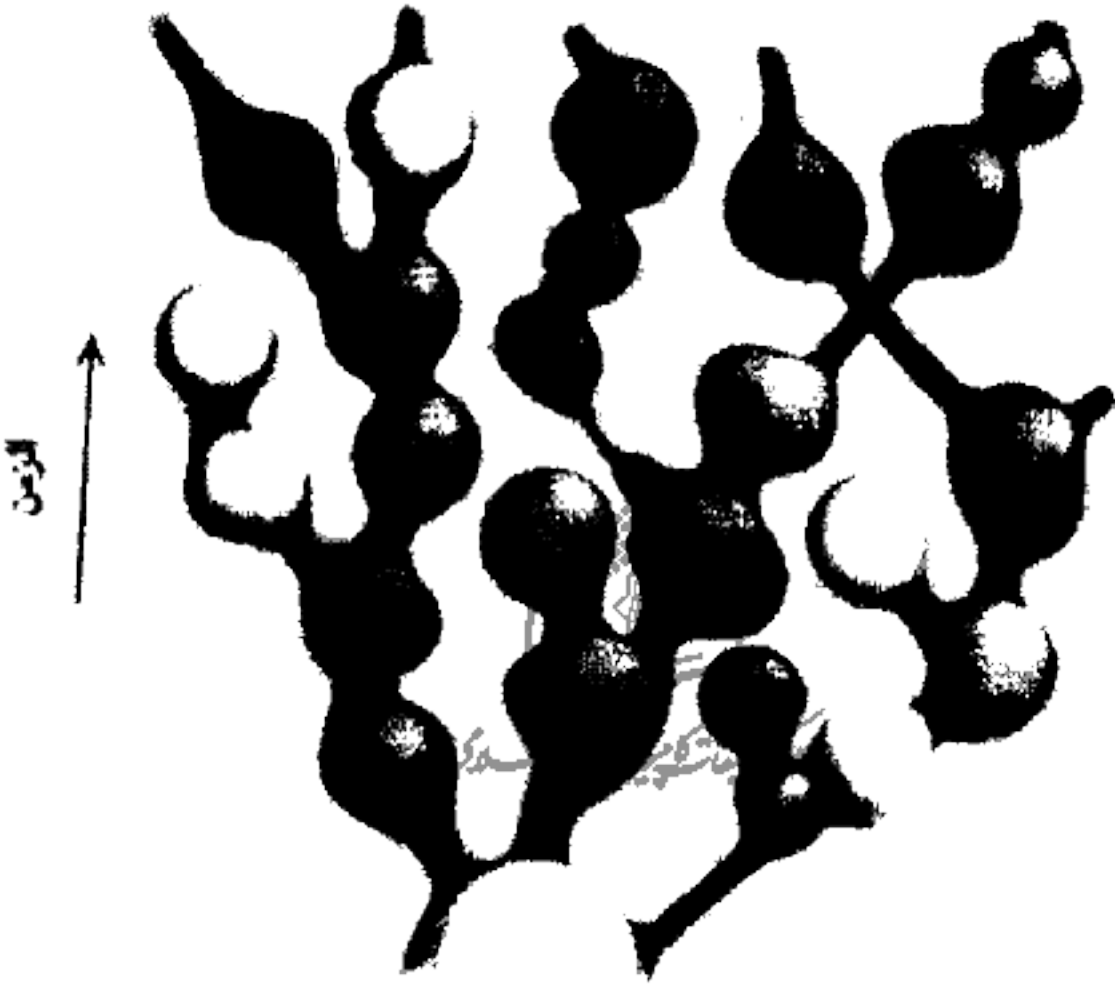
(الشكل ٣٨) يبدو الكون المتجدد ذاتيا على شكل شعب ممتد من الفقائيع التضخمية
