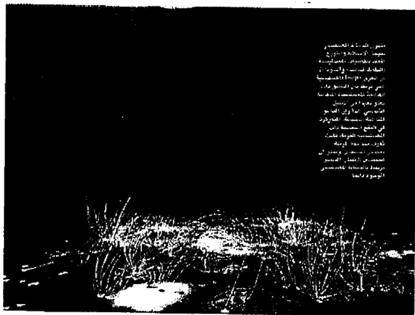
(الشكل ٢٦) التسخين الاكليلي المنتشر وارتباطه بالبساط المغناطيسي الموجود دائما
