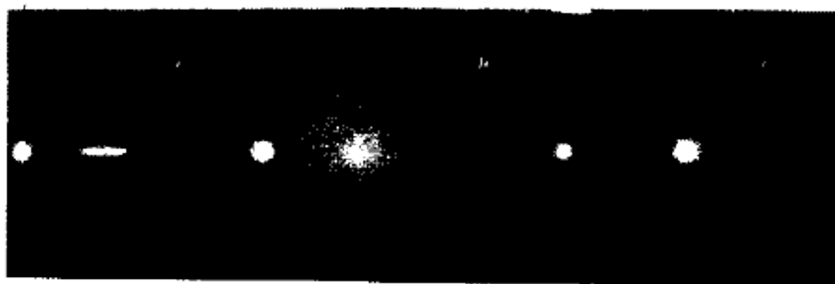
(الشكل ٤٣) الاقزام البيضاء هي الناتج الأخير للتطور النجمي
