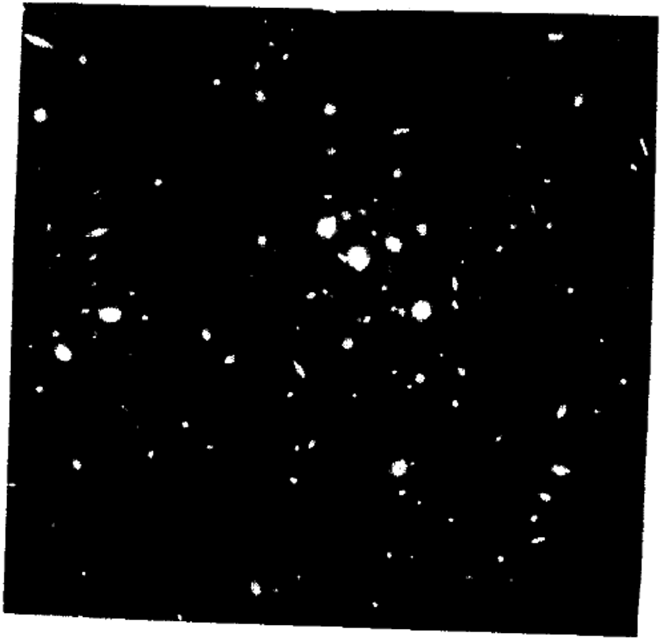
(الشكل ٣٠) التعداد الشاقل والذي تنجم عنه الصور البيضوية الخافتة لمجرة نائية
